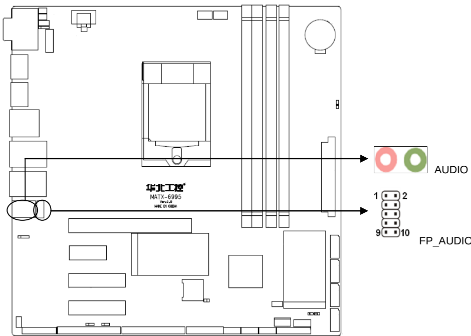
FP_AUDIO:
