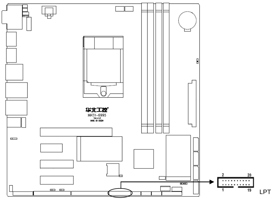
LPT:
