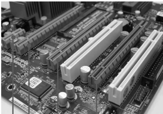
PCIE1-Steckplatz (x1-Modus)
