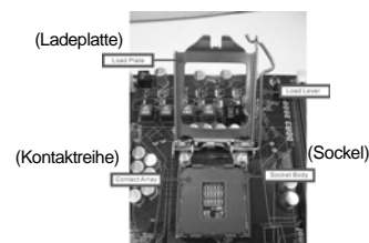
1156-Pin Socket Übersicht
