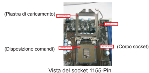
Vista del socket 1155-Pin
