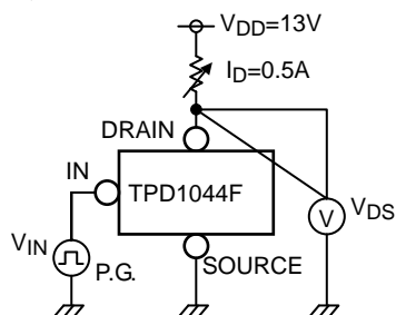
測定回路
