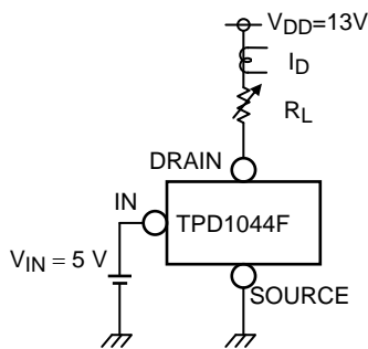
測定回路
