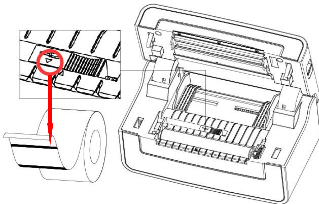
图四（侦测器对准黑标所在位置）
