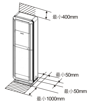
图1 操作空间
