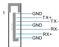
SATA_1/SATA_2/ SATA_3/SATA_4
