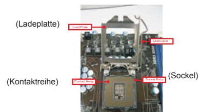
1155-Pin Socket Übersicht
