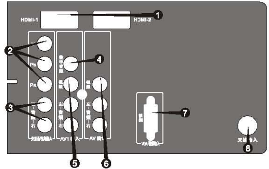
后AV端子示意图
