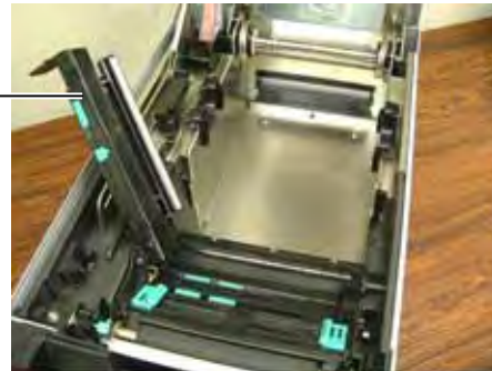
上部探测组件
