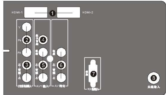
后AV端子示意图
