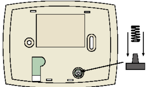
接收器的后部面板
