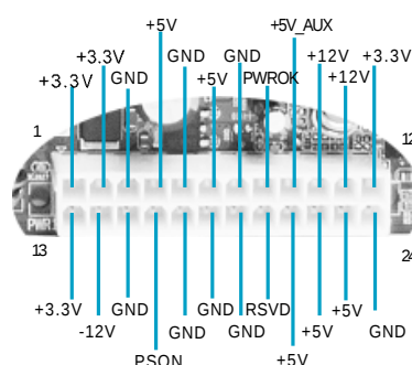
24-pin ATX 电源接头
