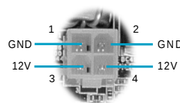
4-pin ATX_12V 电源接头
