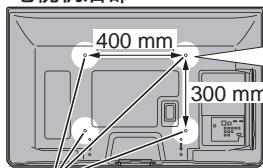
壁挂式支架安装孔
