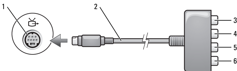
1 S-video 电视输出连接器 2 分量视频适配器 3 S/PDIF 数字音频连接器 * 4 Pr (红色) 分量视频输出连接器 5 Pb (蓝色) 分量视频输出连接器 6 Y (绿色) 分量视频输出连接器
