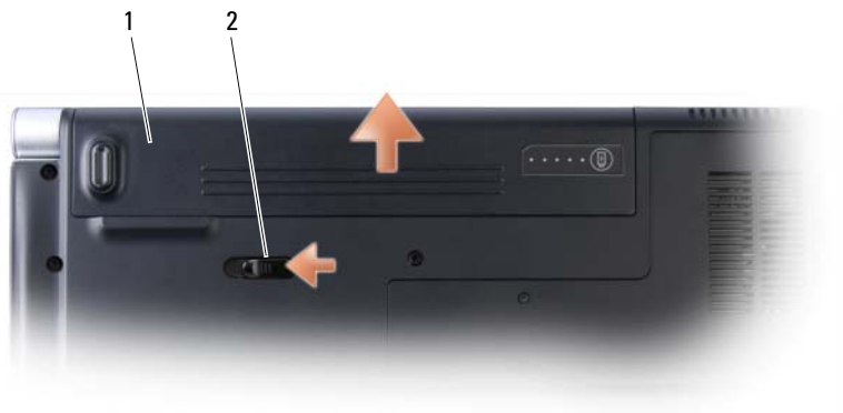
1 电池 2 电池释放门锁
