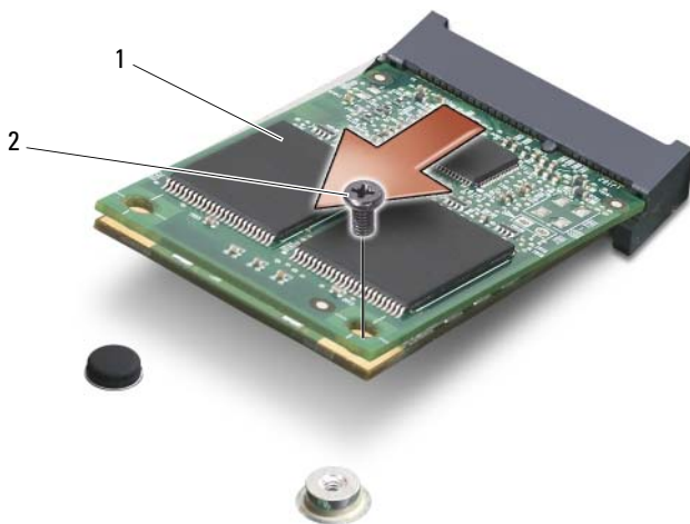
1 FCM 卡 2 M2 x 3 mm 固定螺钉
