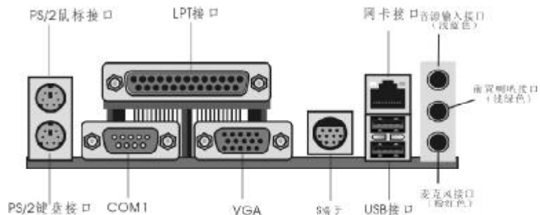
ITX-M4S1LA(-2/3/4)后面板接口 (打印口及S端子为可选)
