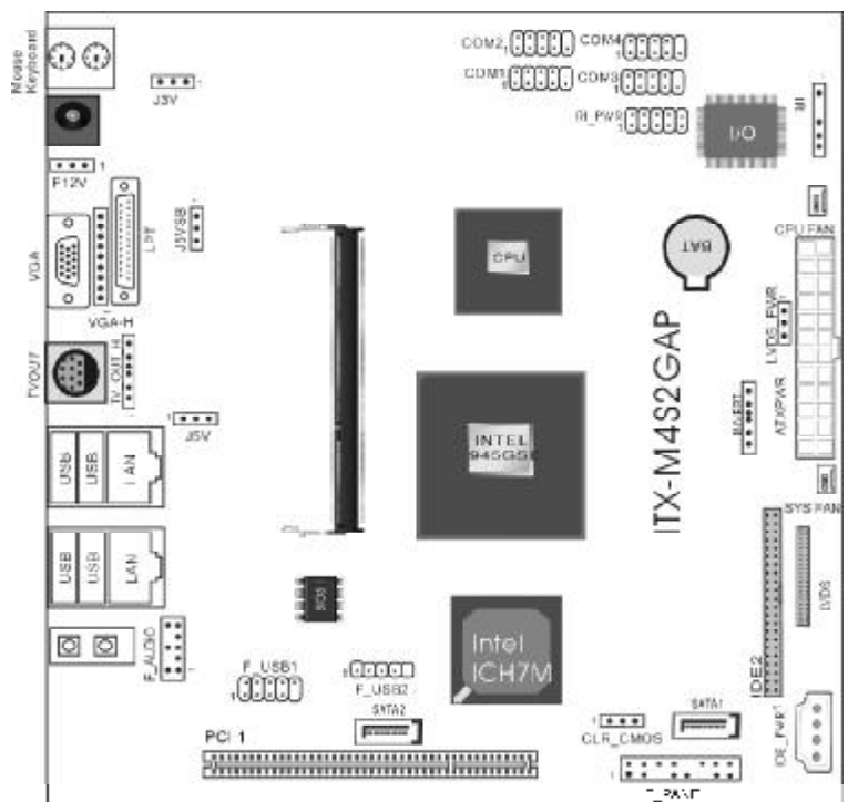
ITX-M4S2GAP 正面图
