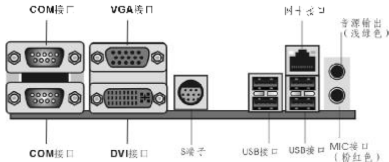
ITX-M4S4DF 后面板接口
