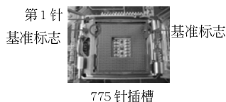
775 针插槽
