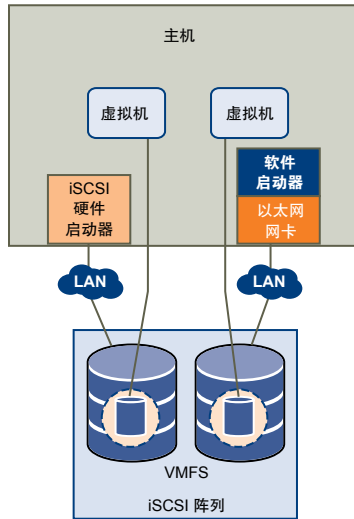
图 8-3 iSCSI 存储器
