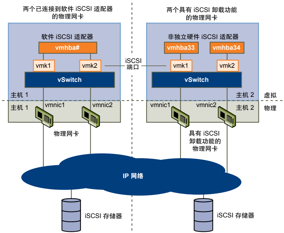
图 6-1 iSCSI 网络
