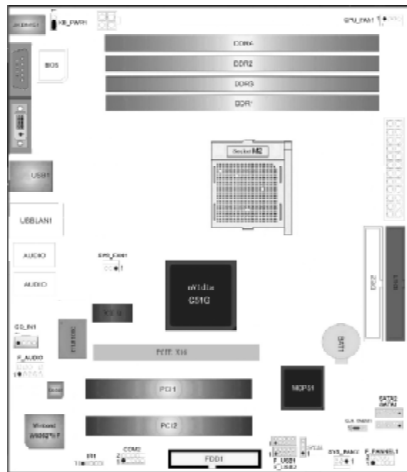
C. NC61- M2 Ver1.5 主机板布局图
