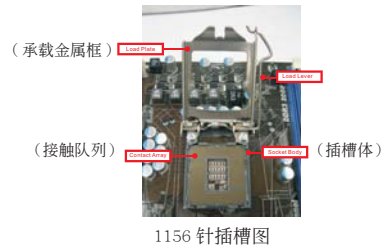
1156 针插槽图
