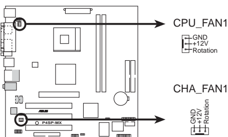
P4SP-MX 12-Volt Cooling Fan Power
