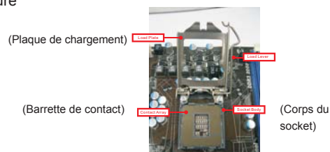
Vue d'ensemble du socket 1155 broches
