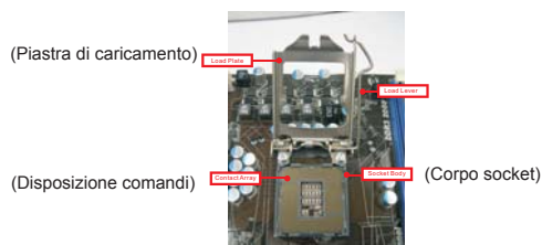
Vista del socket 1155-Pin
