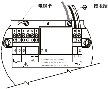
HART接线
