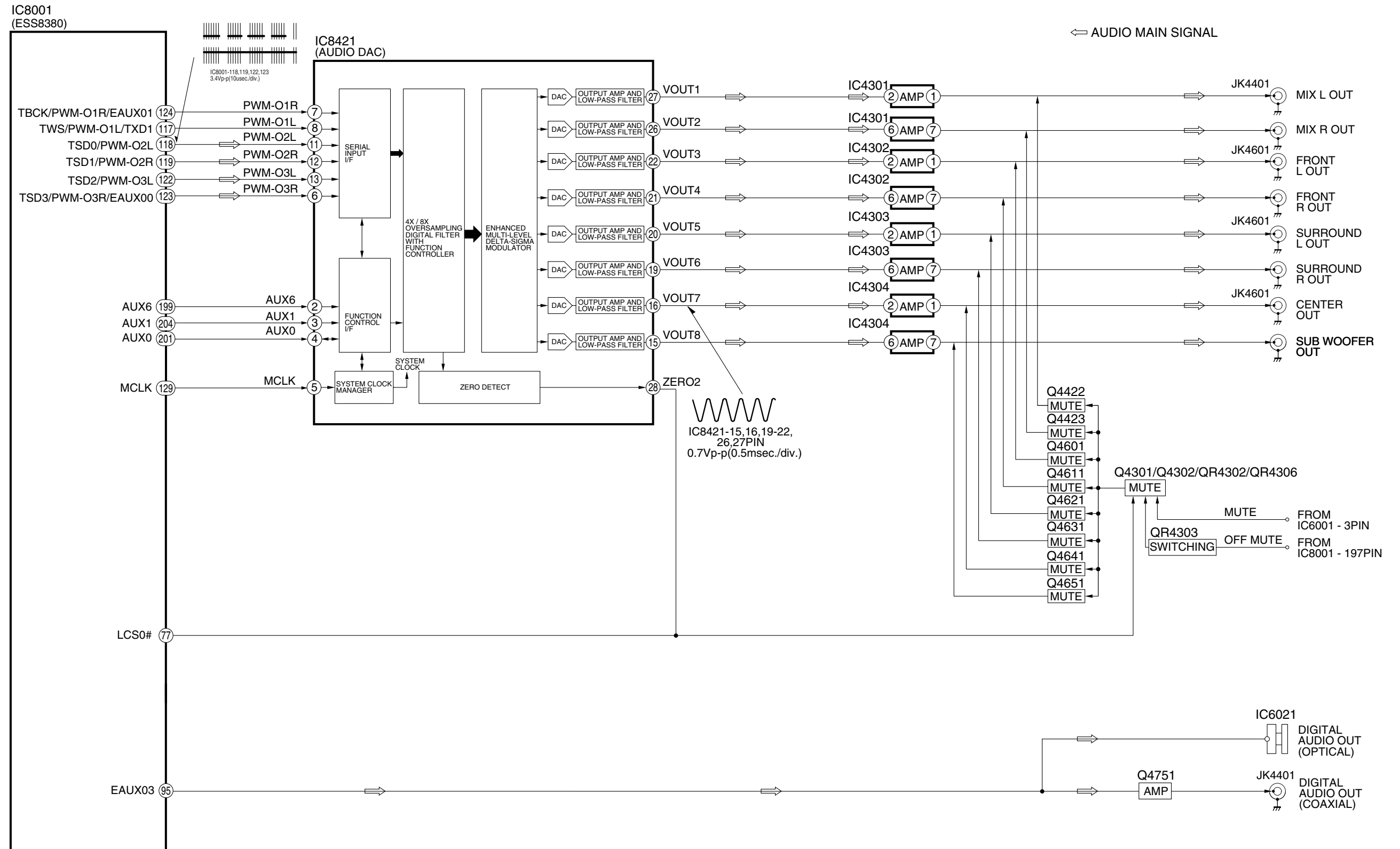
DVD-S830GK/S860GK 音频框图
