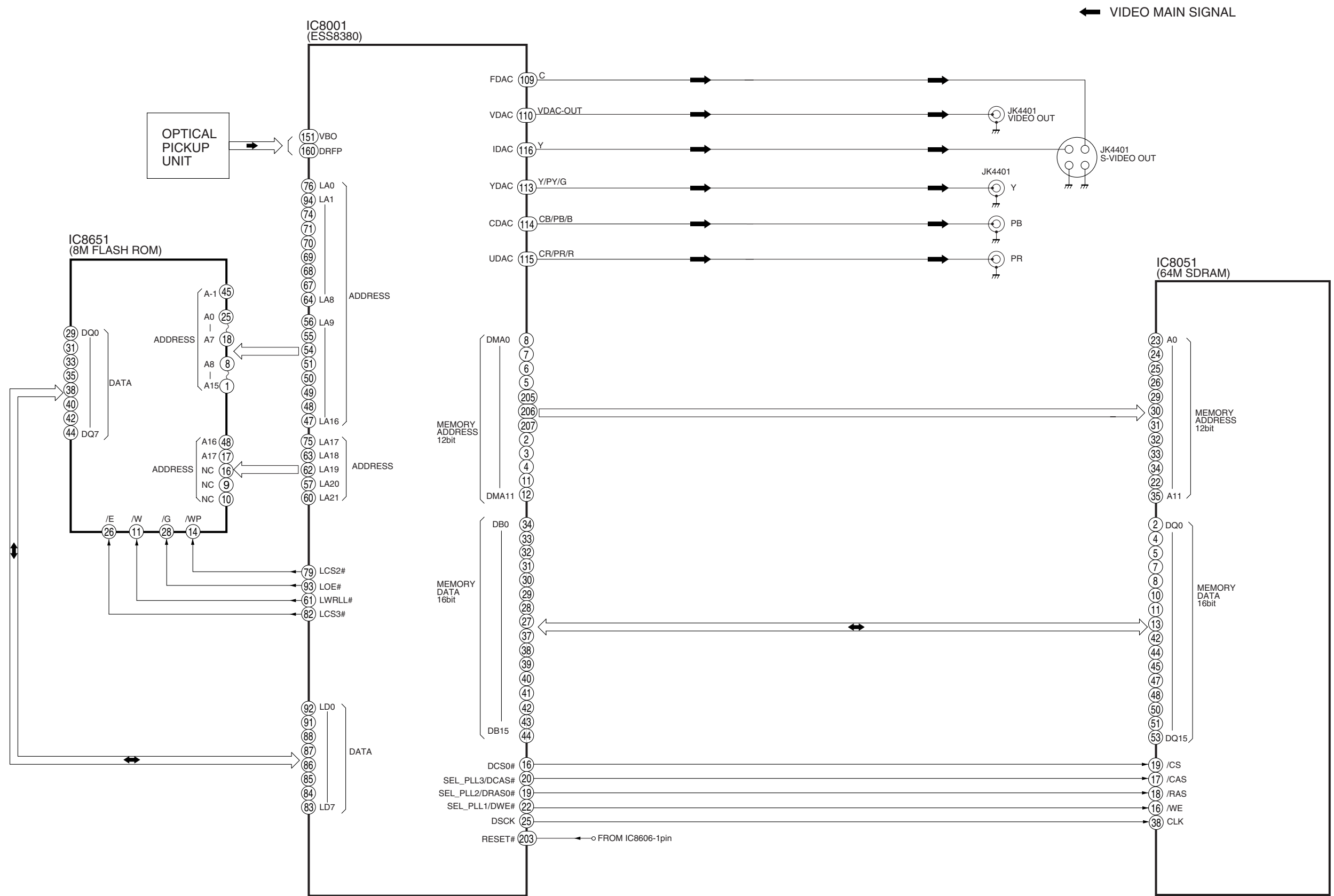
DVD-S830GK/S860GK 视频框图
