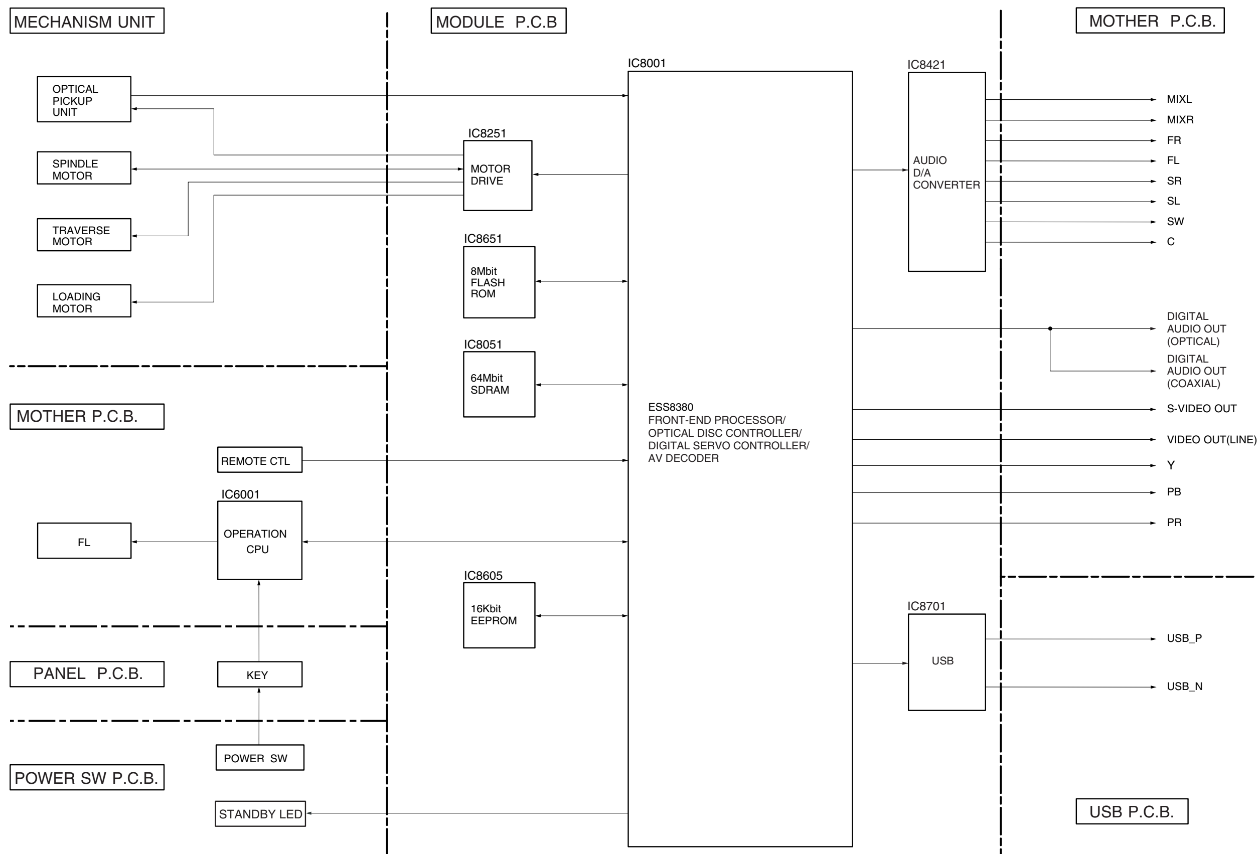
DVD-S830GK/S860GK 总框图
