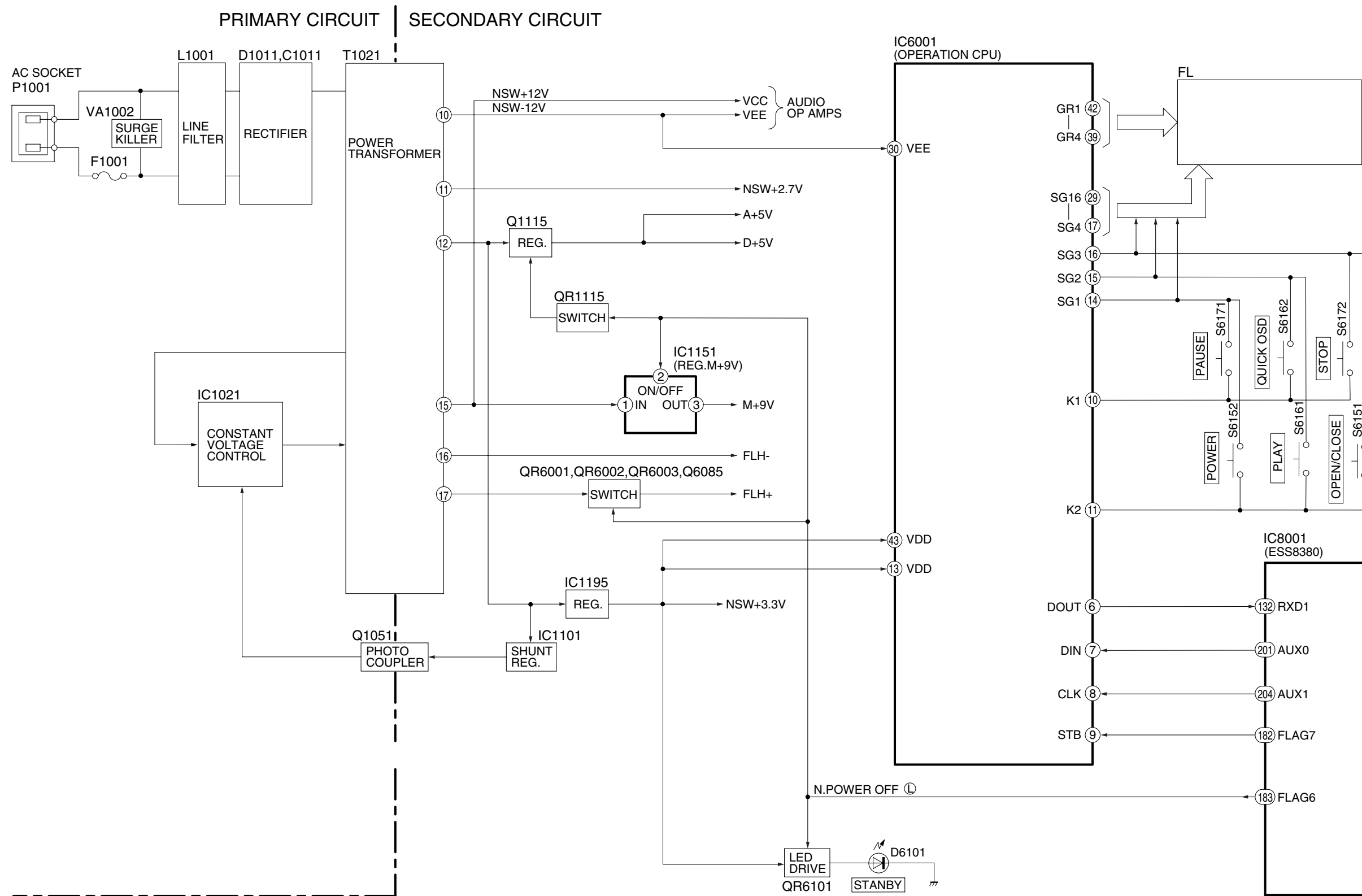
DVD-S830GK/S860GK 电源框图
