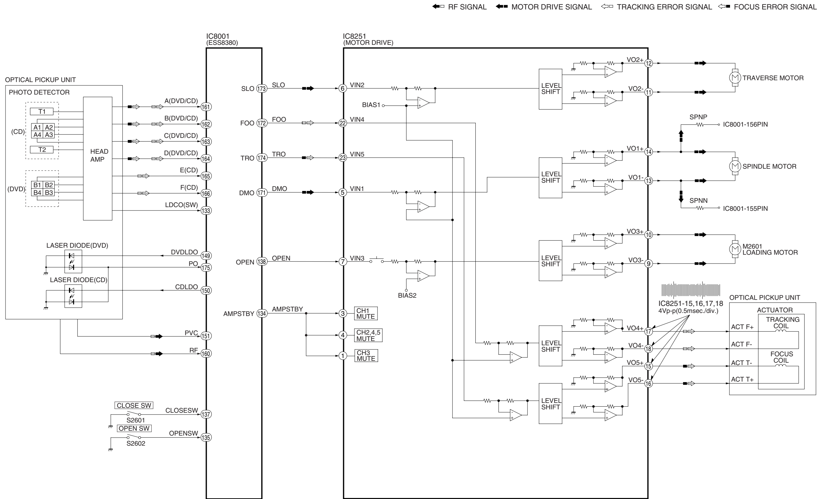
DVD-S830GK/S860GK 伺服框图
