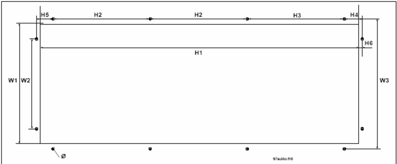
图 5-5. 法兰安装所需开口尺寸, FR7
