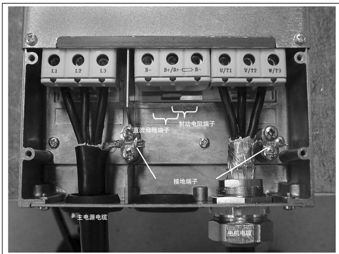
图 6-12. Vacon NX 的电缆安装, FR6
