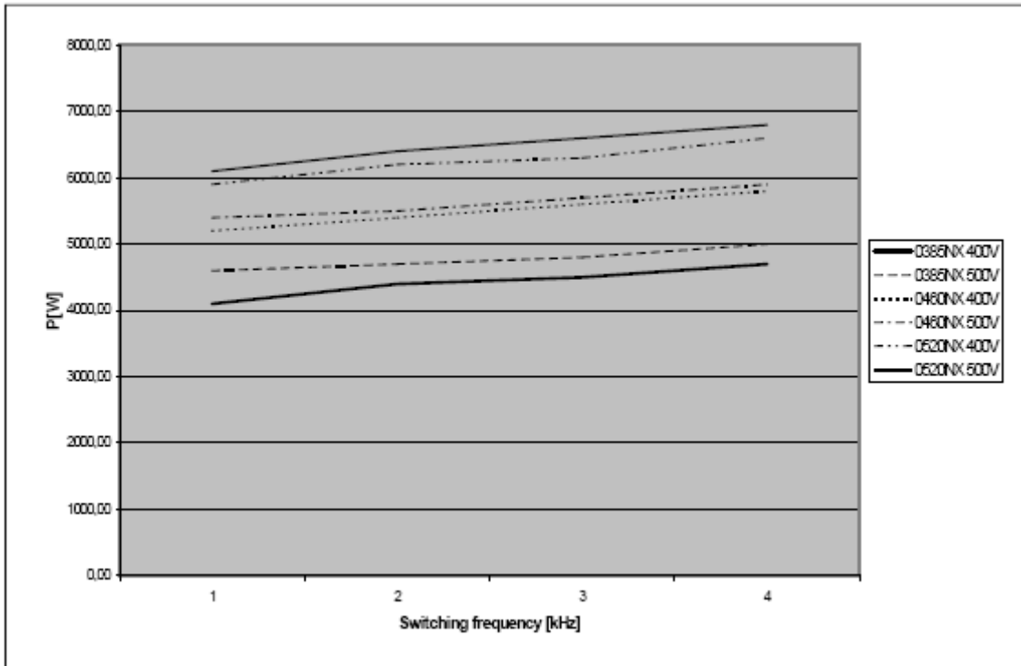
图5-19. 提高斩波频率造成的功率损失, 0385...0520NX5
