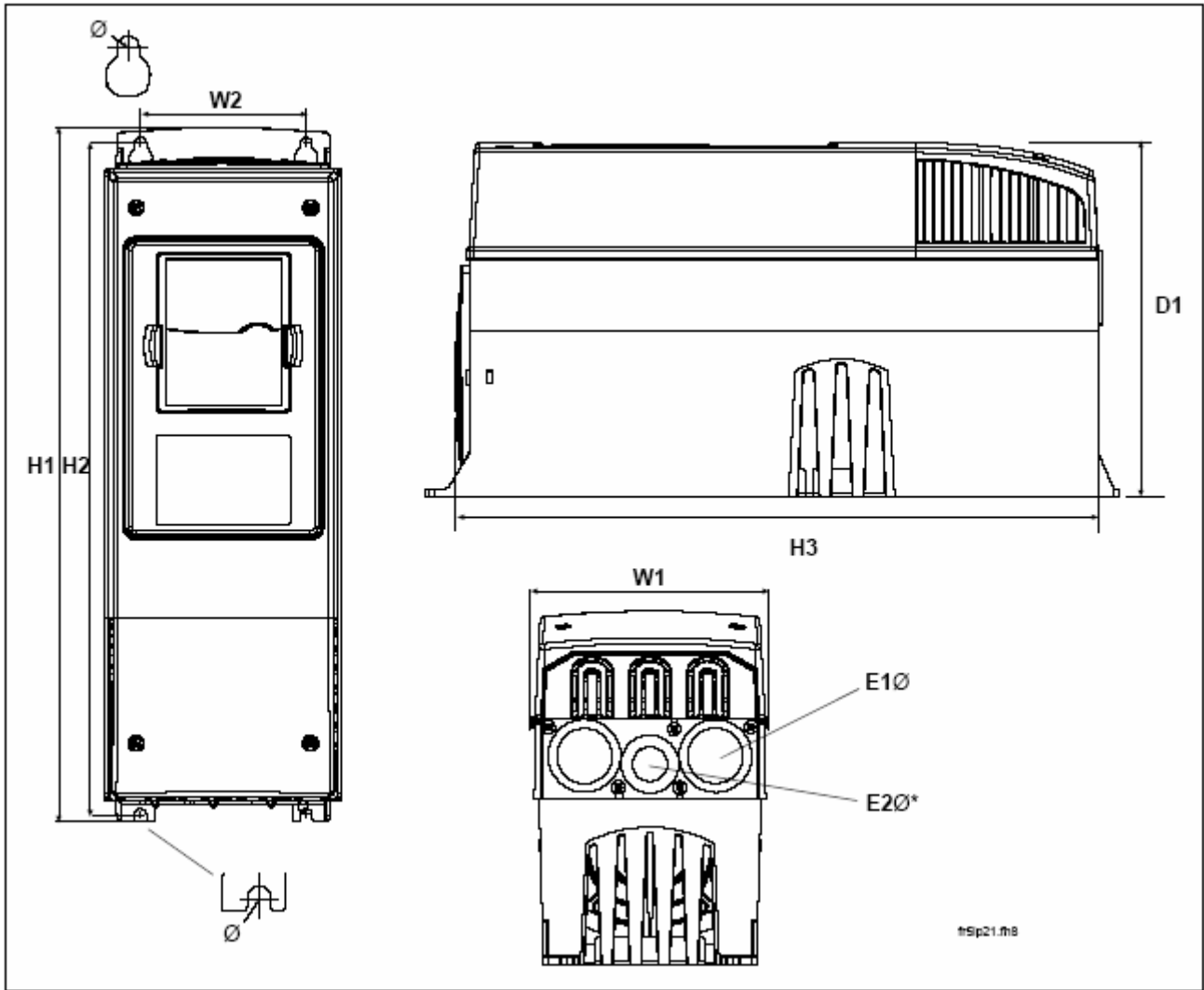
图 5-1. Vacon NX 尺寸
