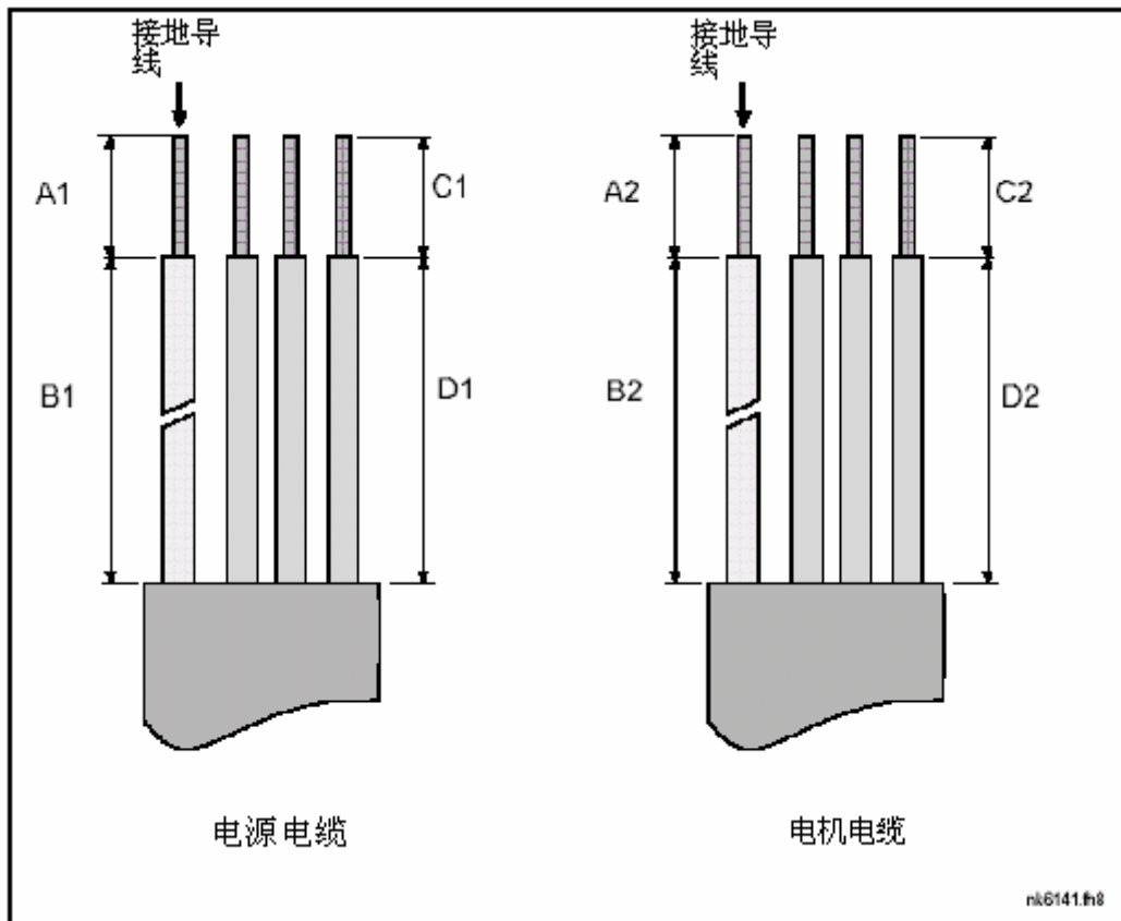
图 6-6. 剥除电缆绝缘层
