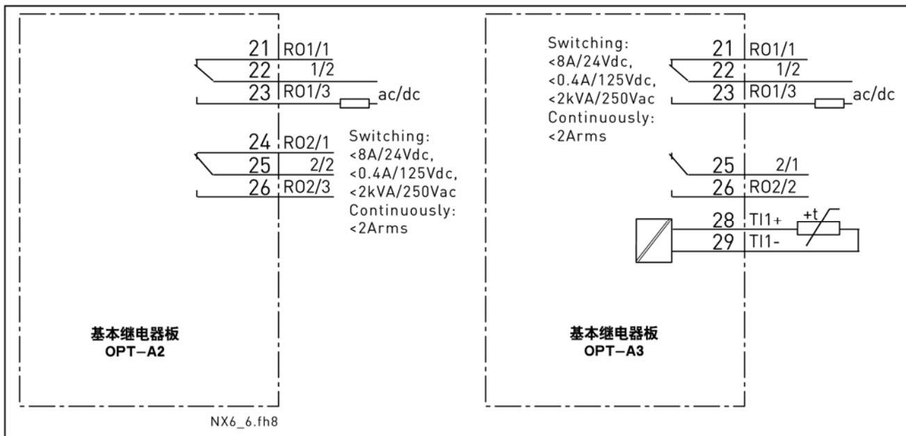
图 6-25. 基本继电器输出板 (OPT-A2/OPT-A3) 的常规接线图
