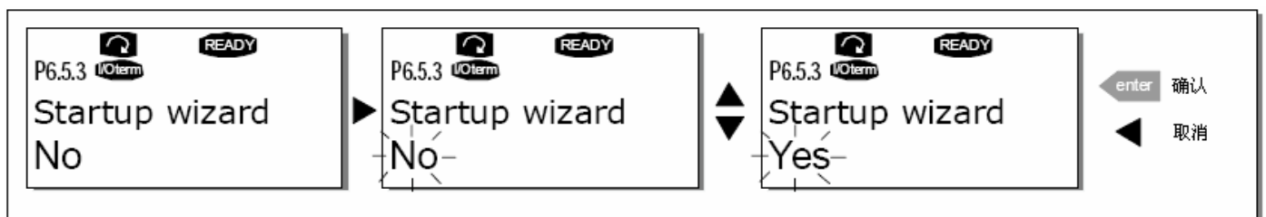
图 7-16. 激活启动向导
