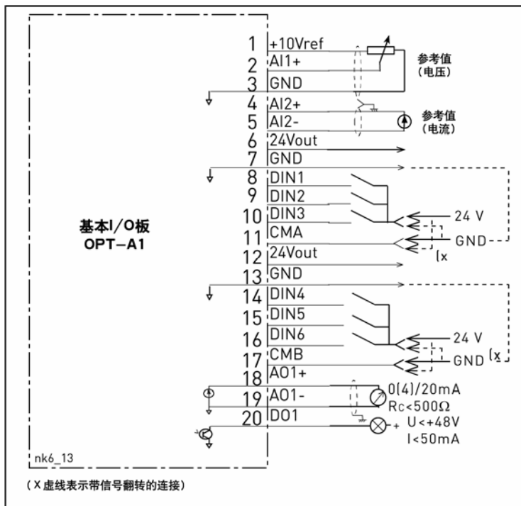
图 6-24. 基本 I/O 板 (OPT-A1) 的常规接线
