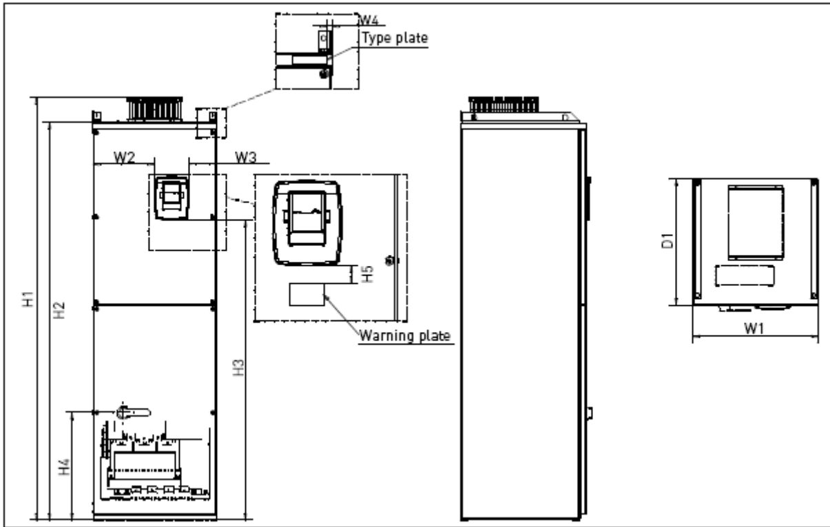
图 5-9. FR10 和 FR11 变频器（立式单元）的尺寸
