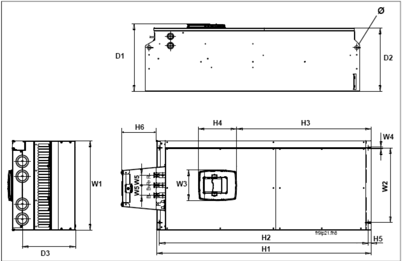
图 5-7. FR9 变频器的尺寸
