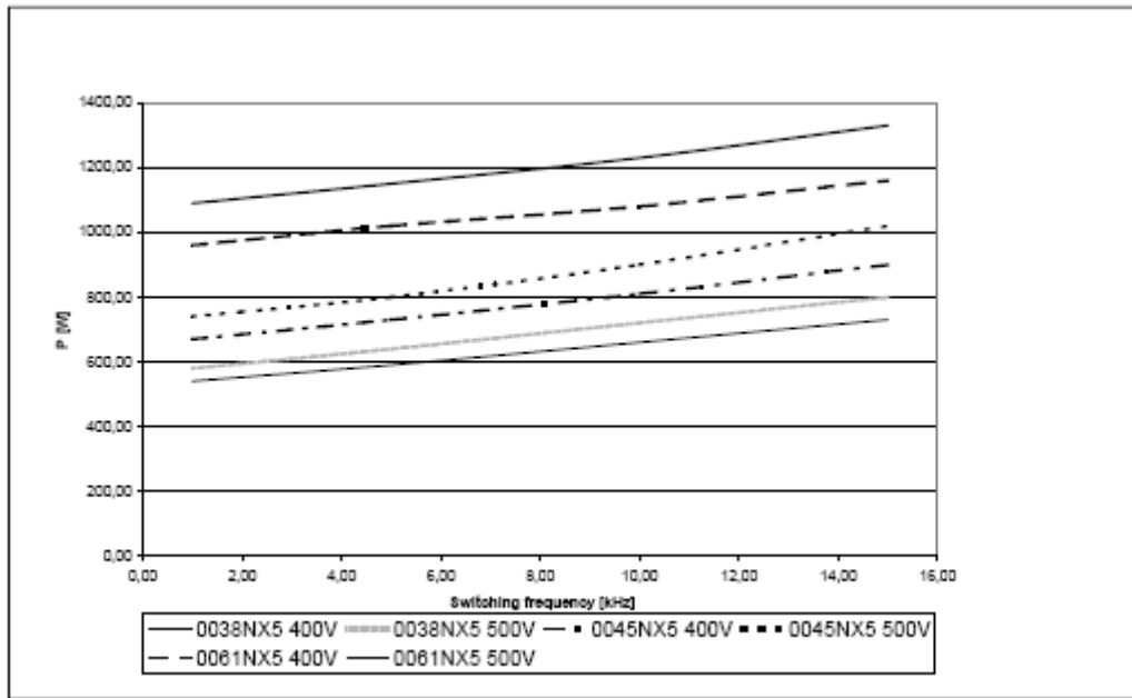
图5-15. 提高斩波频率造成的功率损失, 0038...0061NX5
