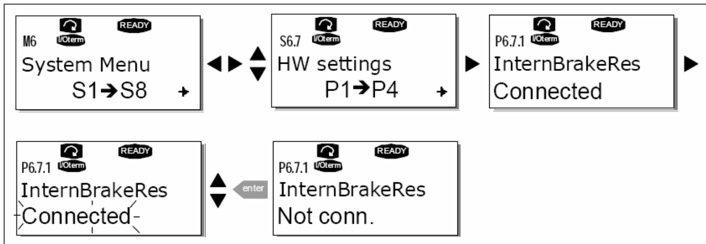
图 7-21. 内部制动电阻的连接
