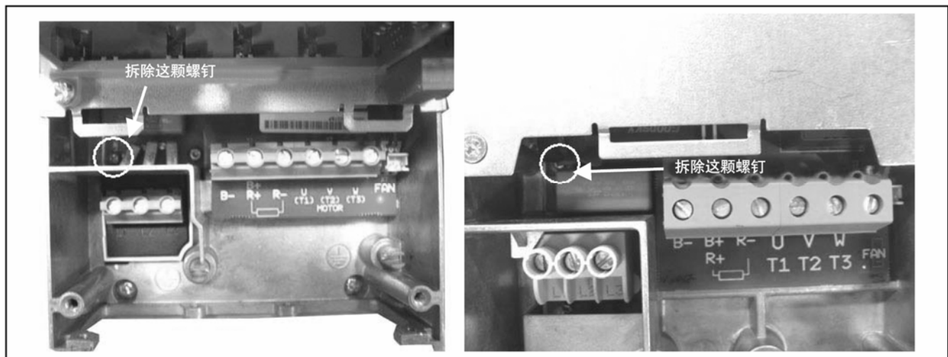
图6-2. 改变EMC防护等级，FR4（左）/FR5（右），首先应拆下电缆盖
