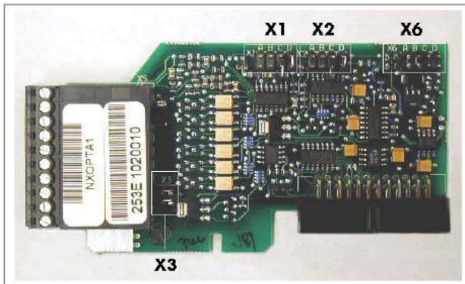
图 6-28. OPT-A1 板上的跳线块
