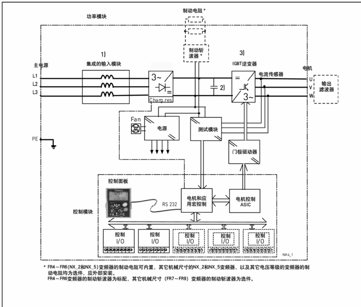
图 4-1. Vacon NX 框图
