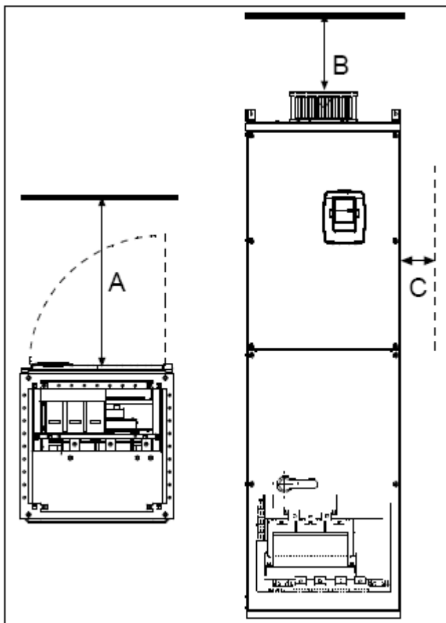
图 5-12. 安装空间
