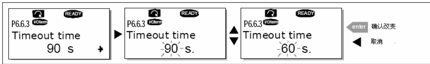
图 7-20. 溢出时间设置
