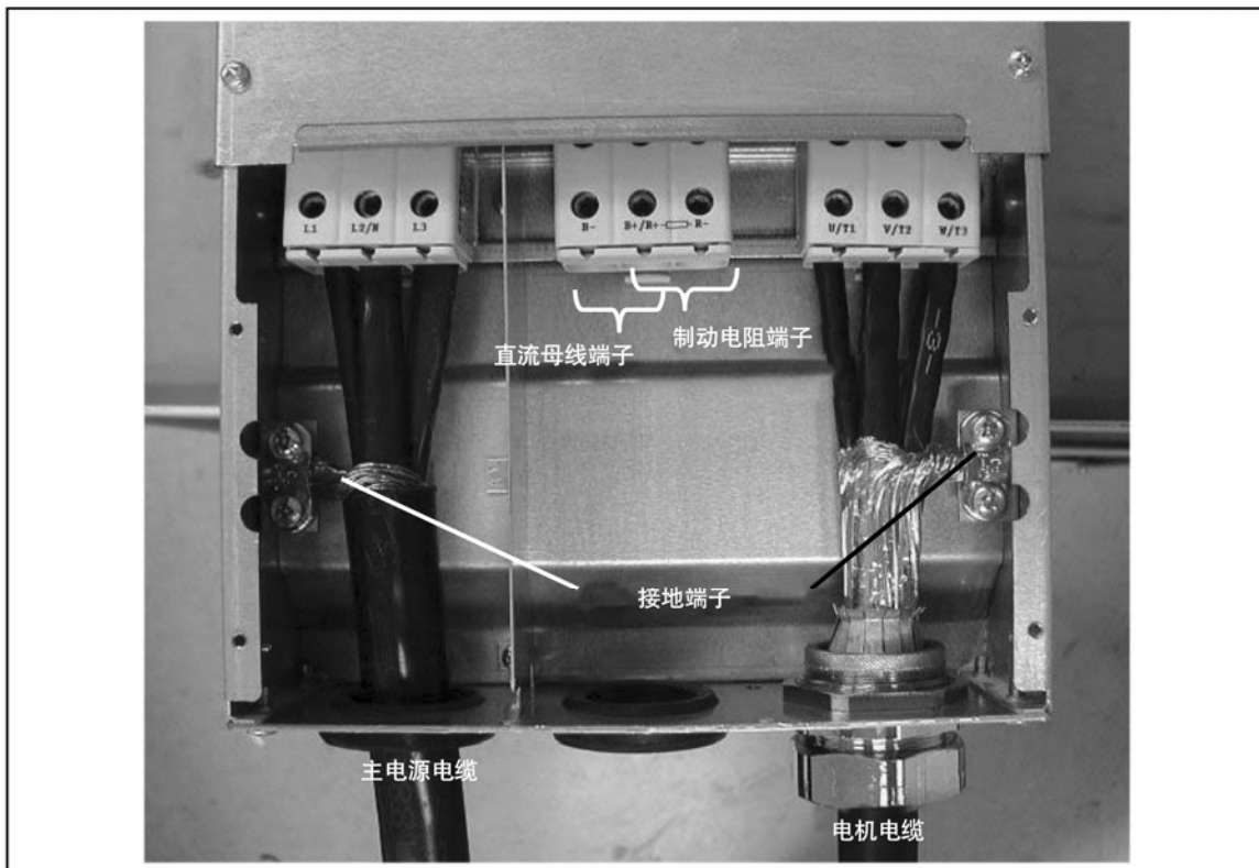
图 6-14. Vacon NX 的电缆安装, FR7
