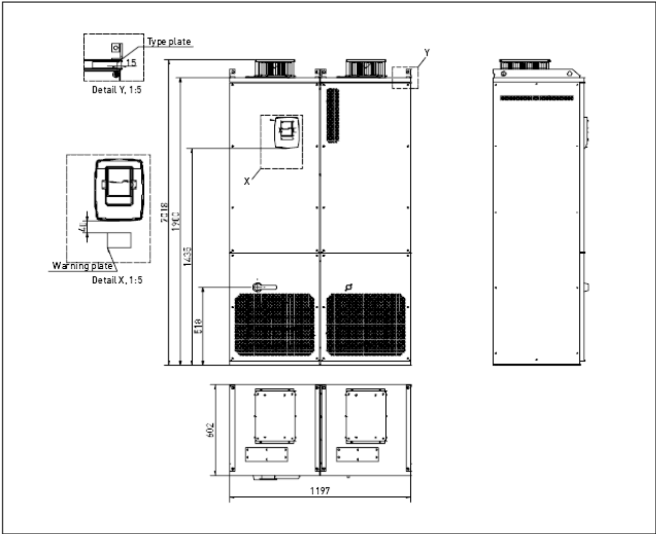
图 5-10. FR12 变频器（立式单元）的尺寸
