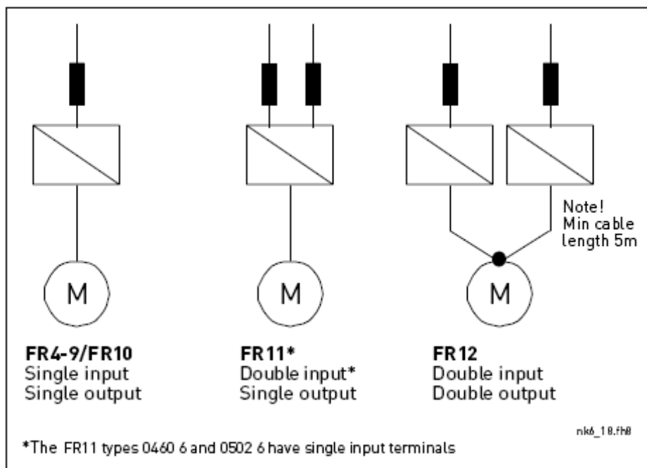
图6-1. FR4 – FR12变频器的功率单元接线原理
