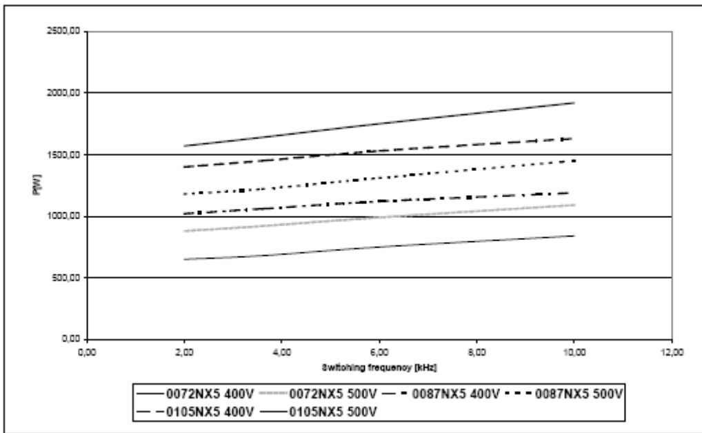
图 5-16. 提高斩波频率造成的功率损失, 0072...0105NX5
