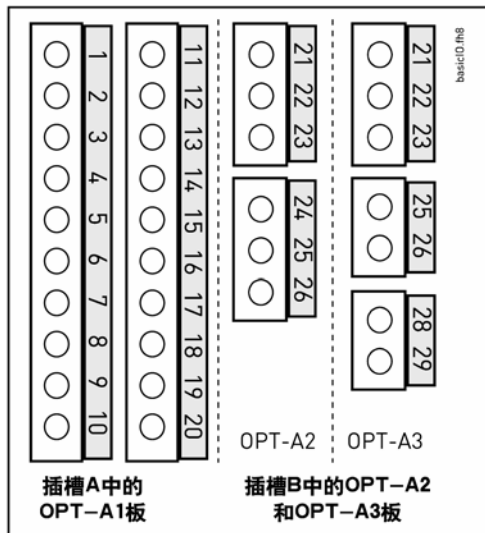
图 6-23. 两块基本板的 I/O 端子
