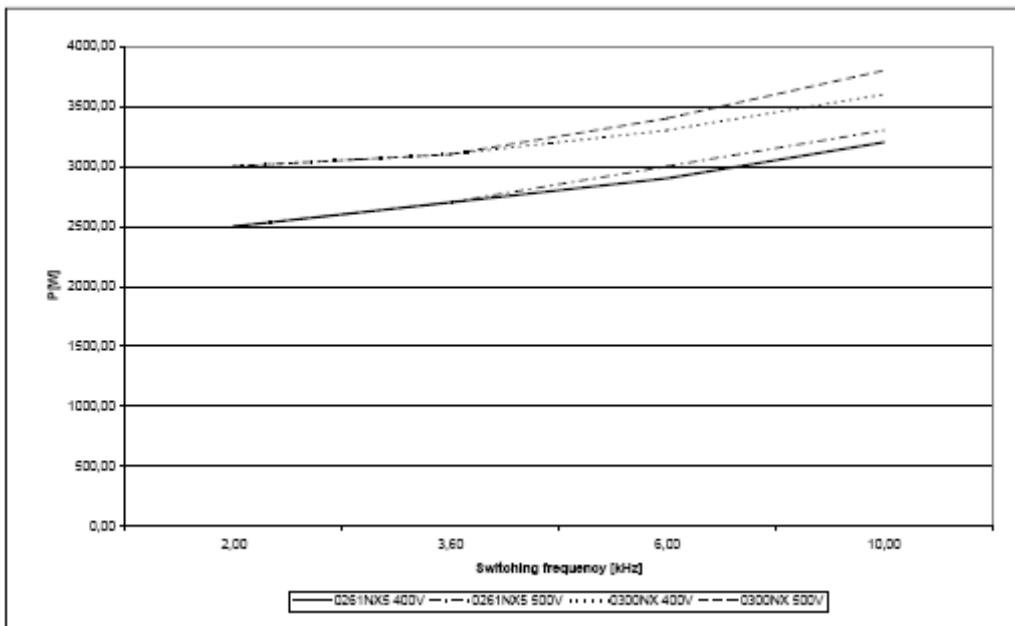
图 5-18. 提高斩波频率造成的功率损失, 0261...0300NX5
