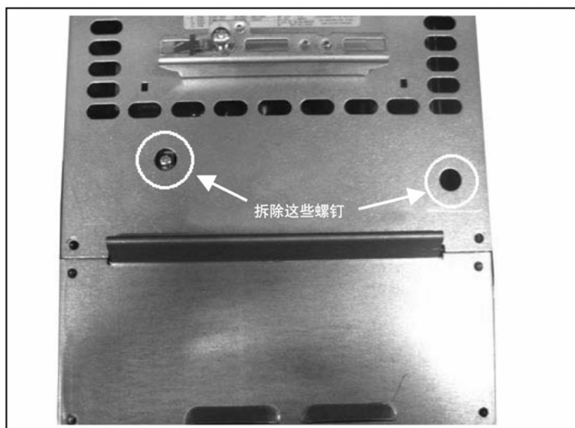
图6-3. 改变EMC防护等级，FR6，无需拆下电缆盖
