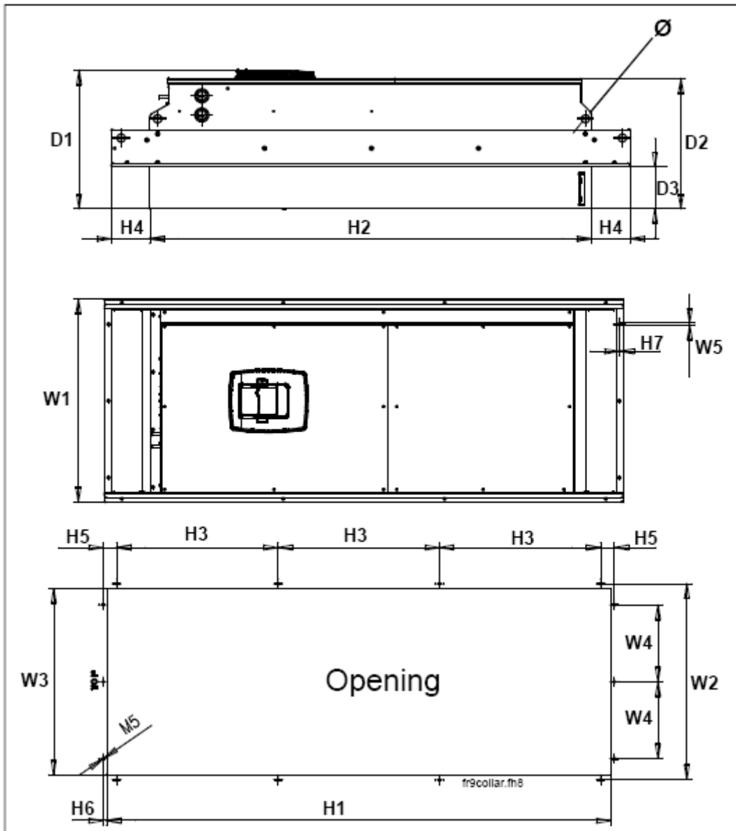
图 5-8. FR9 变频器的尺寸，法兰安装
