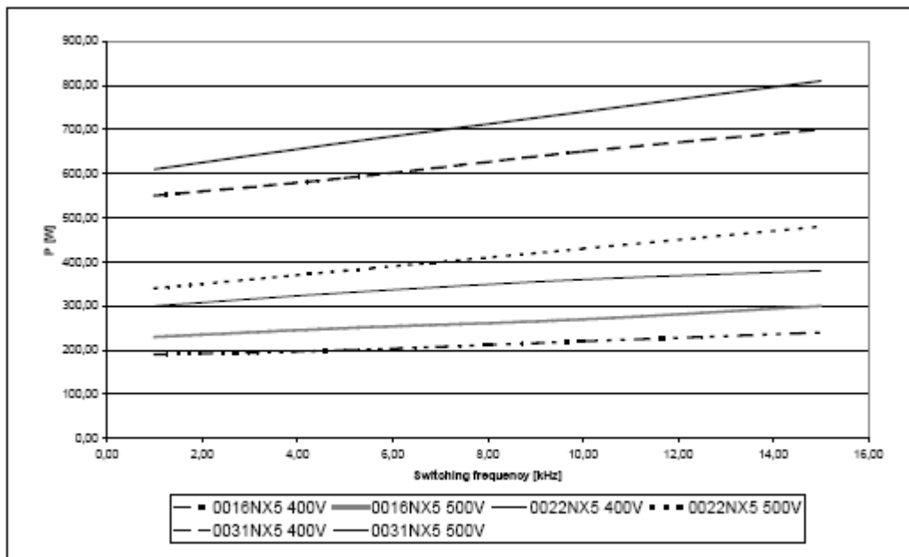
图 5-14. 提高斩波频率造成的功率损失, 0016...0031NX5
