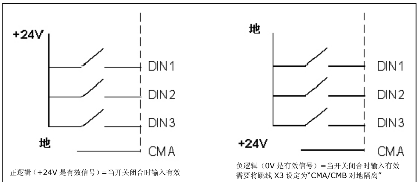
图 6-27. 正/负逻辑
