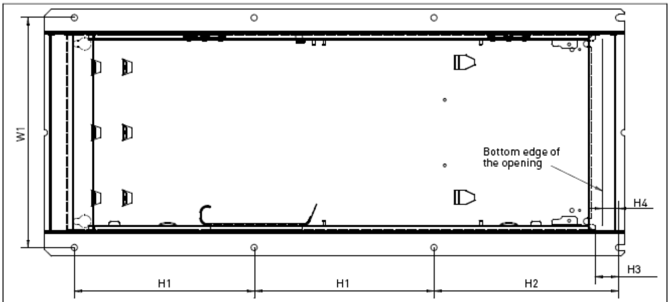
图 5-6. 法兰安装所需开口尺寸, FR8
