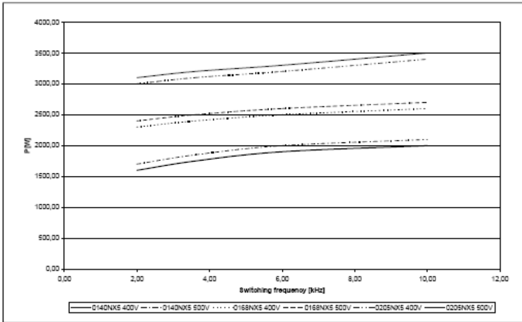
图 5-17. 提高斩波频率造成的功率损失, 0140...0205NX5
