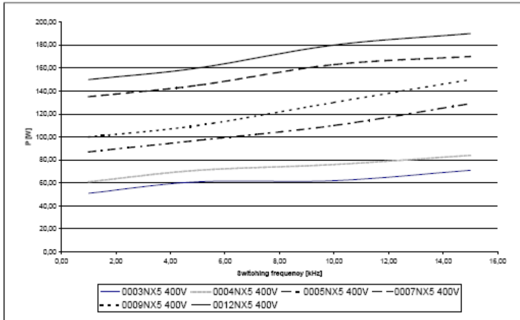
图 5-13. 提高斩波频率造成的功率损失, 0003...0012NX5
