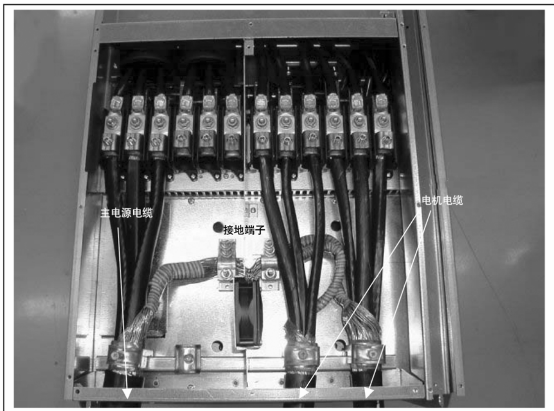
图 6-19. Vacon NX 的电缆安装, FR9
