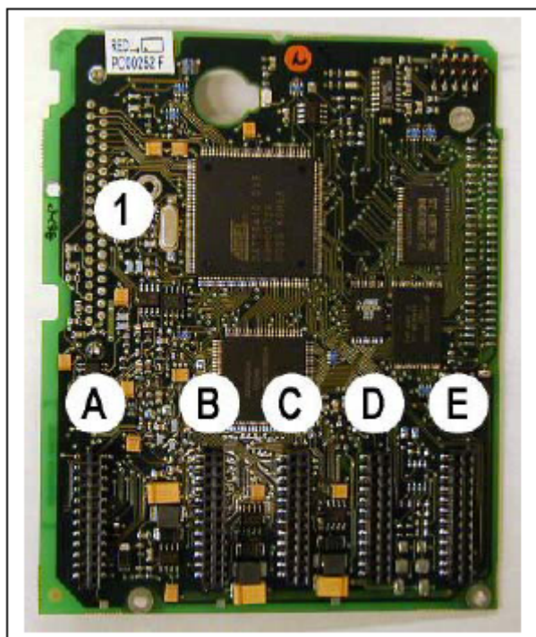
图 6-21. Vacon NX 的控制板
