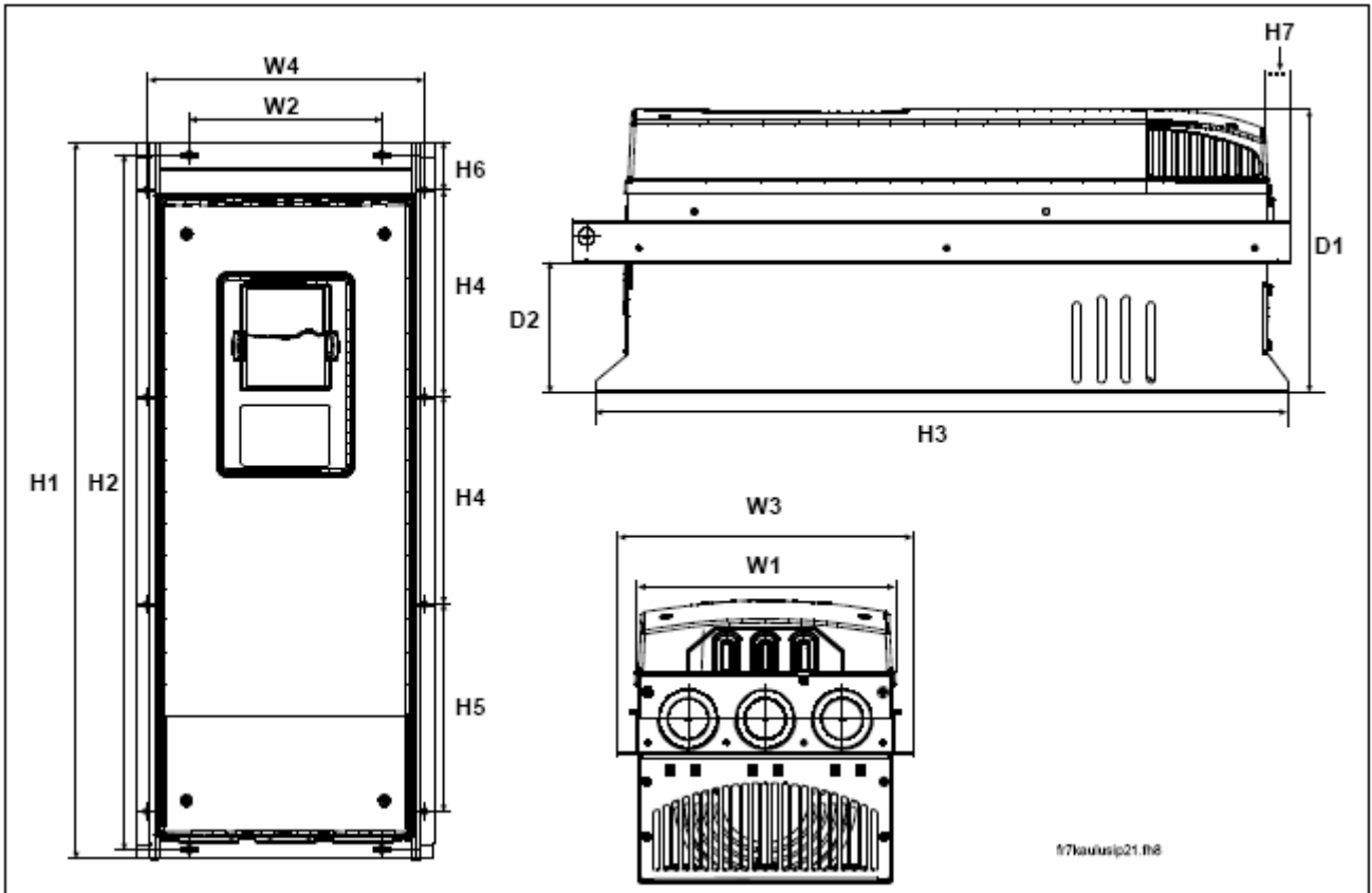
图 5-4. FR7 和 FR8 变频器的尺寸，法兰安装
