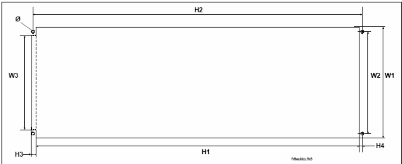
图 5-3. 法兰安装所需开口尺寸, FR4—FR6
