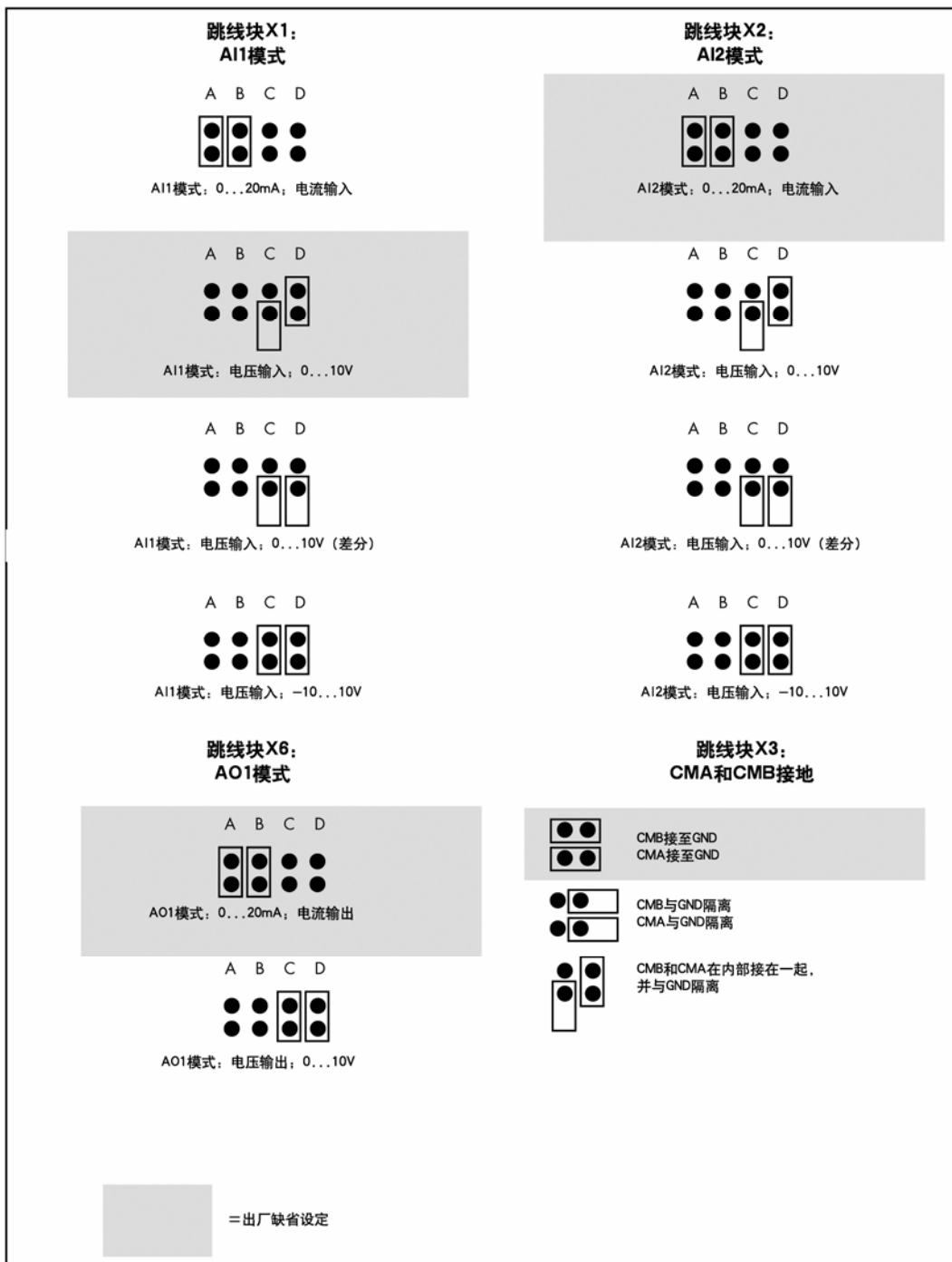
图 6-29. OPT-A1 板上的跳线选择
