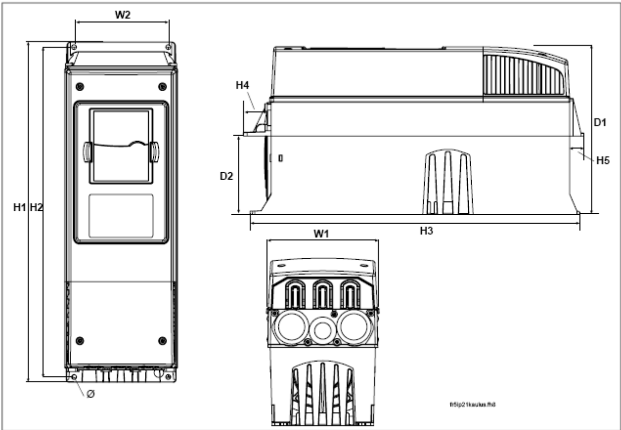
图 5-2. Vacon NX 尺寸, FR4—FR6, 法兰安装
