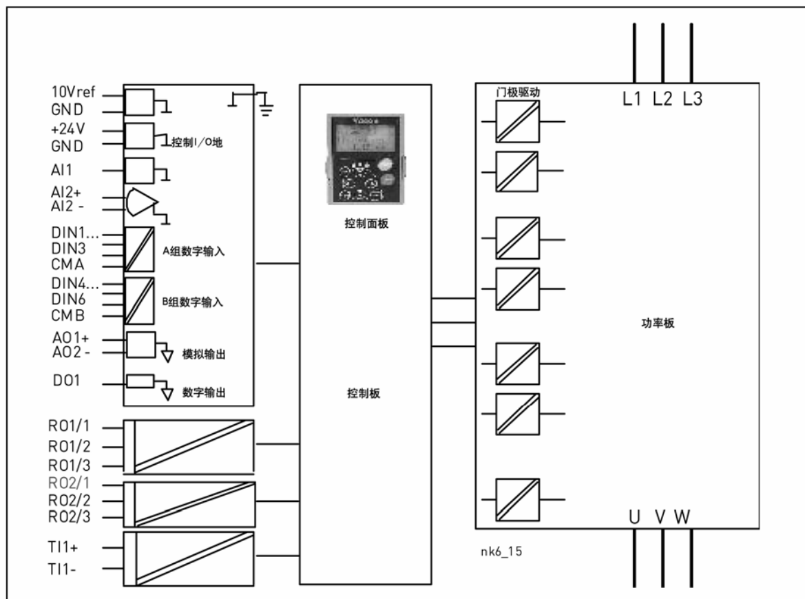
图 6-26. 电隔离
