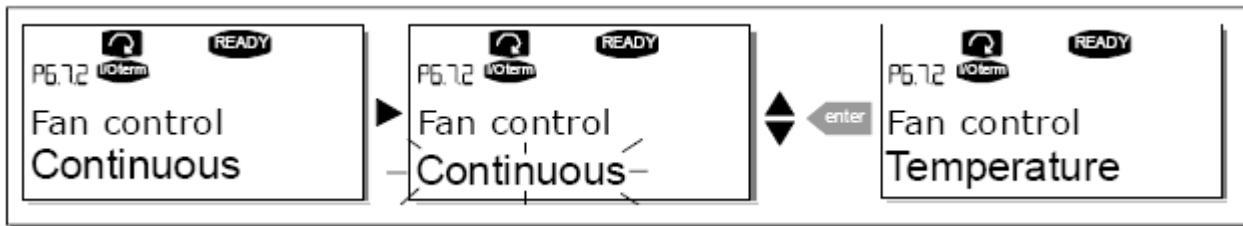
图 7-22. 风扇控制功能
