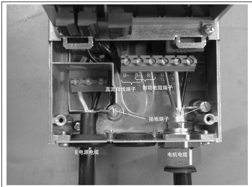
图 6-8. Vacon NX 的电缆连接, FR4
