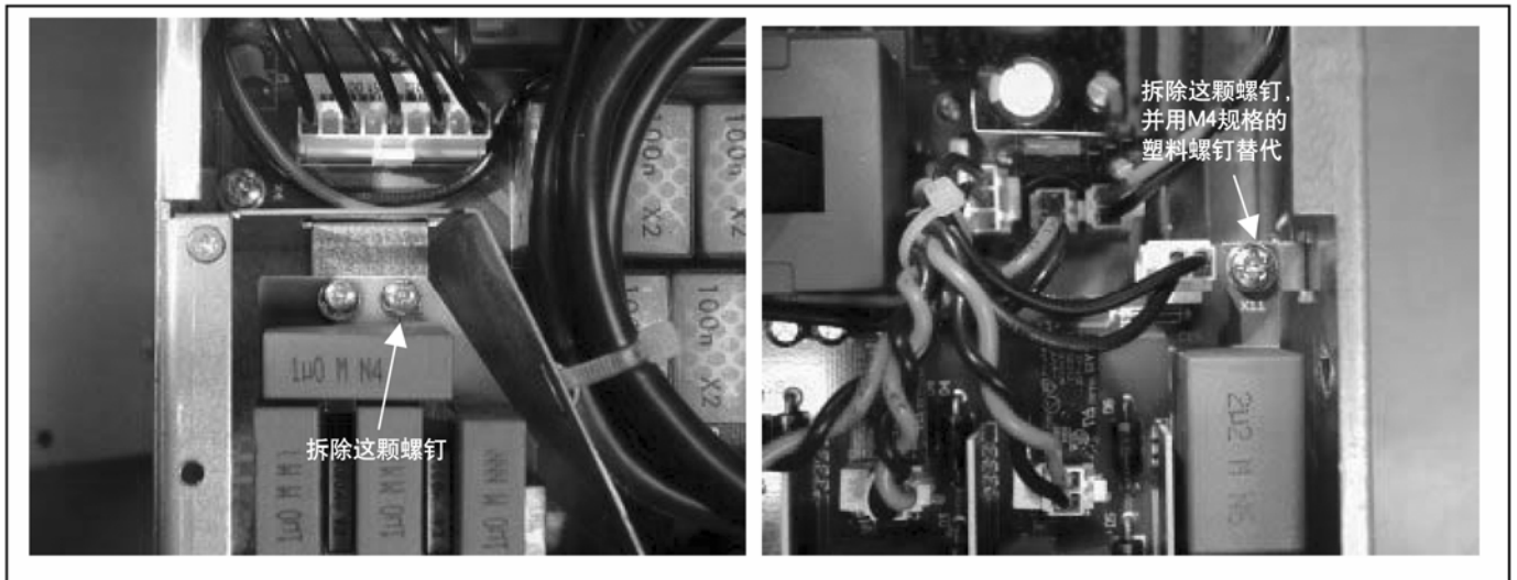
图6-4. 改变EMC防护等级, FR7
