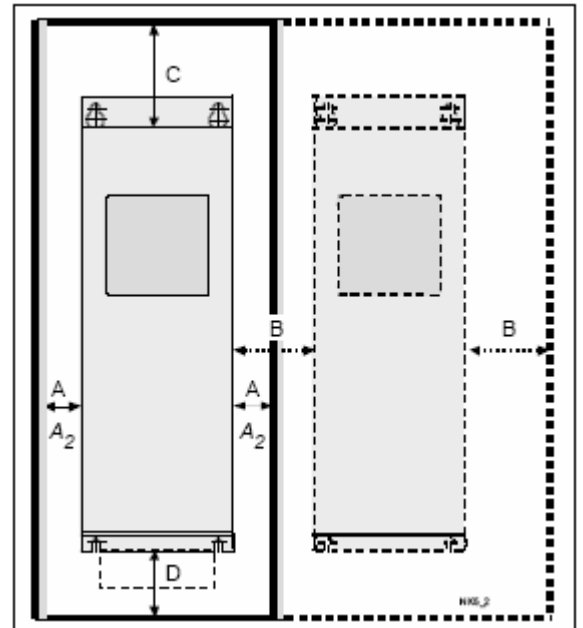
图 5-11. 安装空间
