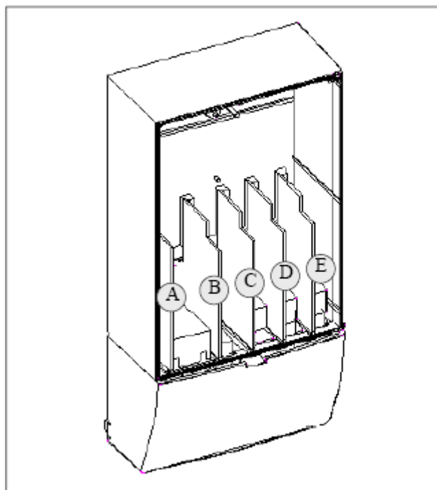
图 6-22. Vacon NX 的基本板和选件板与控制板的连接
