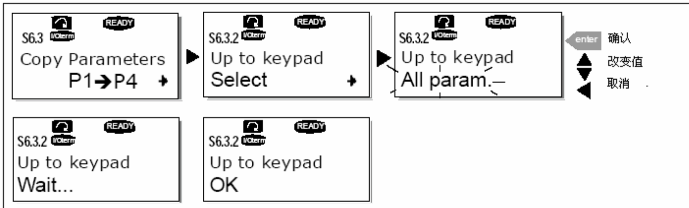
图 7-12. 上传参数到控制面板
