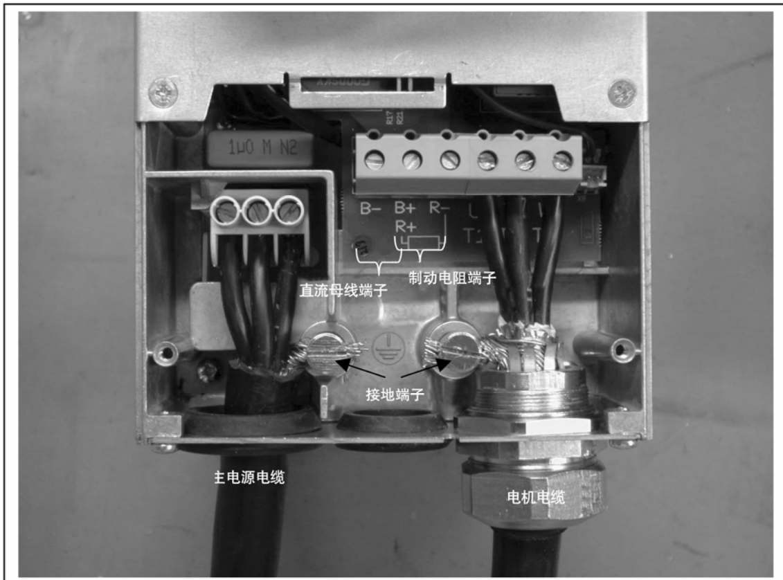
图 6-10. Vacon NX 的电缆安装, FR5
