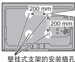
壁挂式支架的安装插孔
