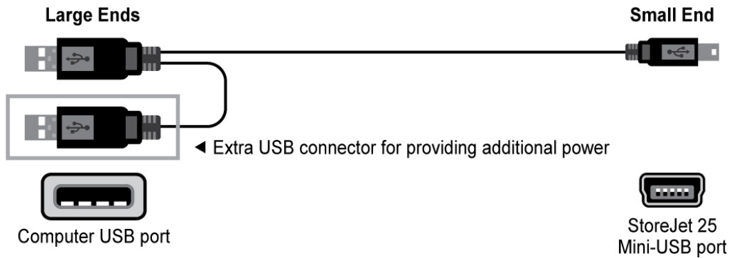
图 2: Mini USB 转 USB A 型连接线 (USB Y 型连接线)
