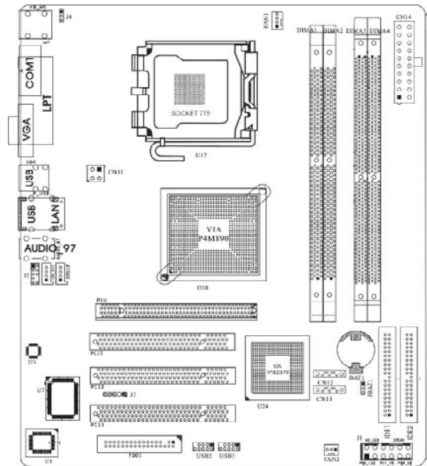
C.M9PV- D Ver2.1 布局图
