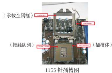
1155 针插槽图
