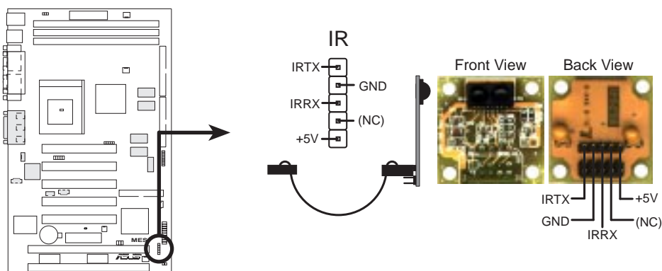
MES Infrared Module Connector
