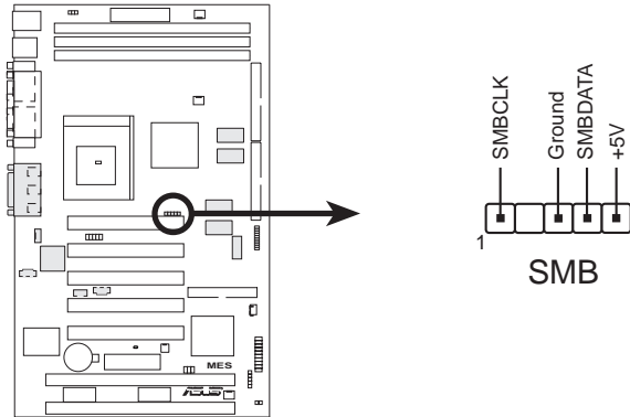
MES SMBus Connector
