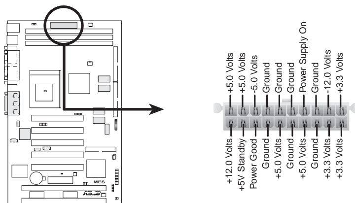
MES ATX Power Connector
