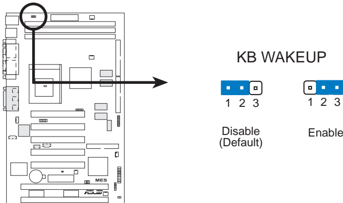
MES Keyboard Wake Up
