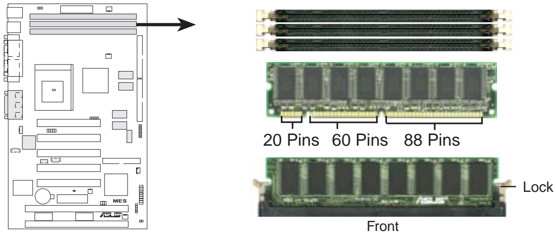
MES 168-Pin DIMM Sockets
