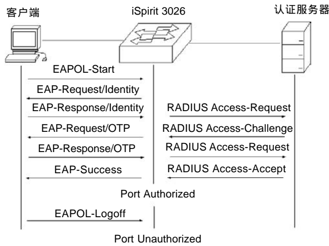
图 8-4 客户端发起认证的协议交互
