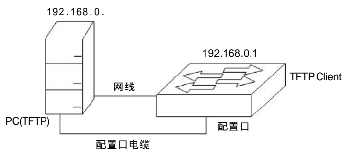
图 1-4 搭建 TFTP 升级环境
