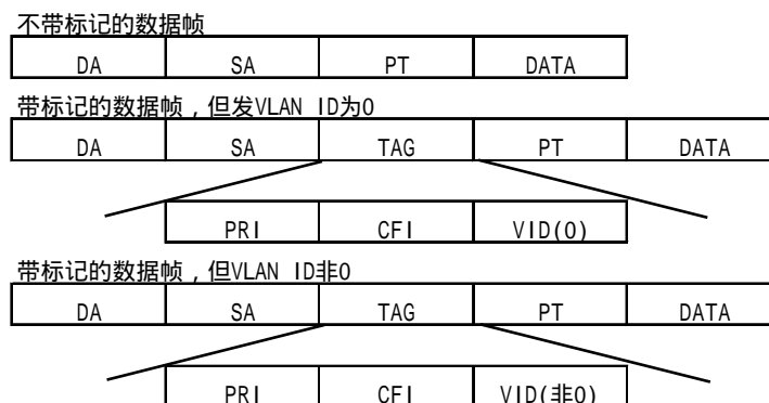
图 3-1 三种不同的数据帧格式
