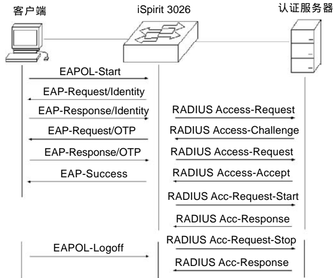
图 8-7 协议流交互
