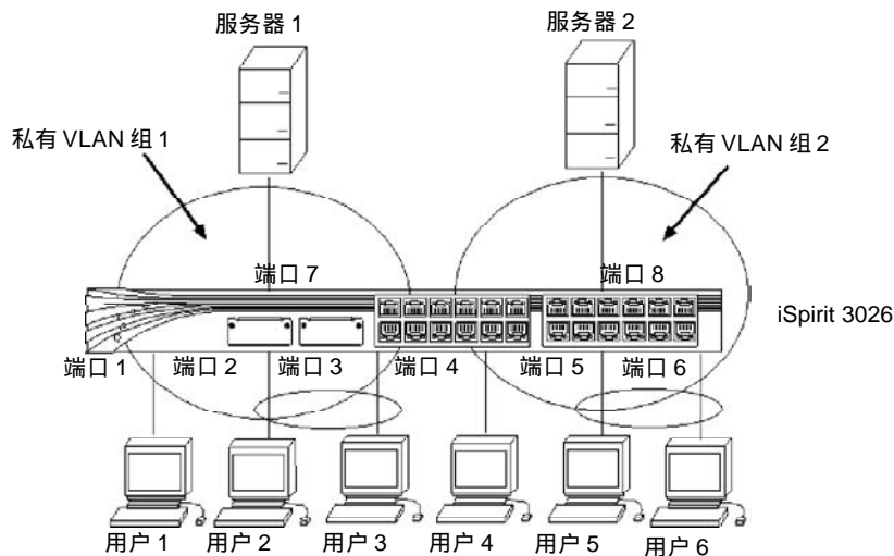
图 4-2 两个私有 VLAN 组
