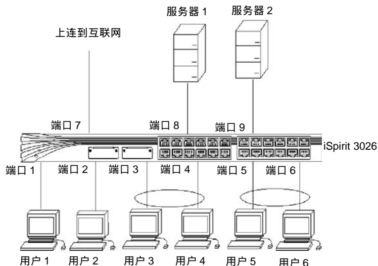
图 4-3 一个私有 VLAN 组
