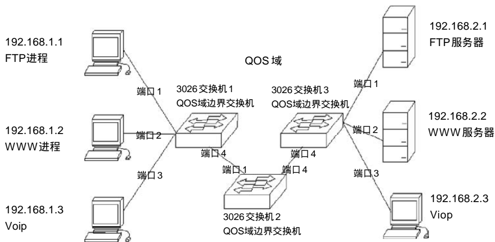
图 12-10 配置 QoS 案例
