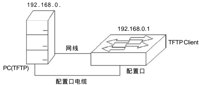
图 1-1 搭建 TFTP 环境
