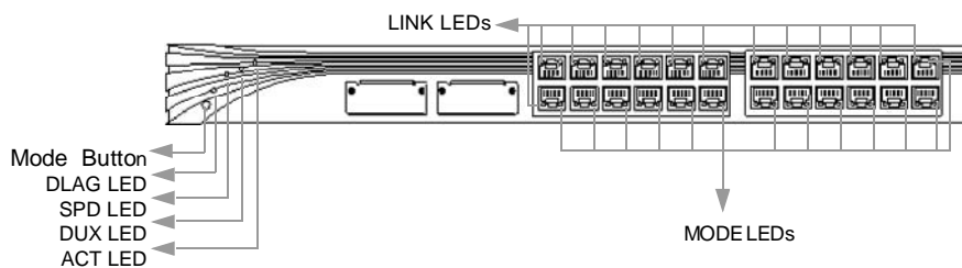
图 1-4 3026 交换机 LED 状态指示灯、模式键和端口 LED 状态指示灯位置图
