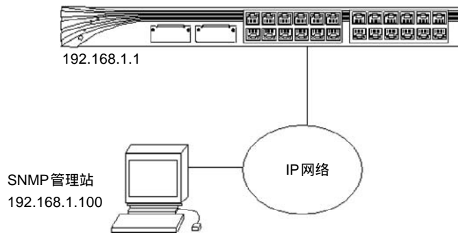
图 9-2 MAC 绑定示例
