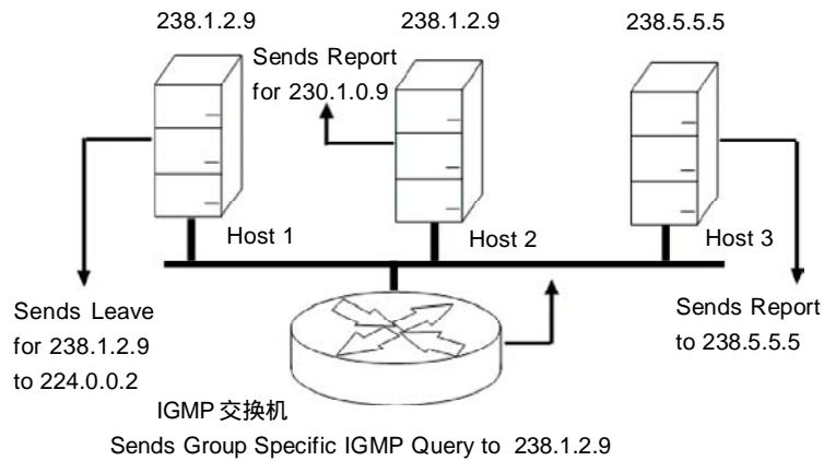
图 14-6 离开组的 IGMP 协议过程
