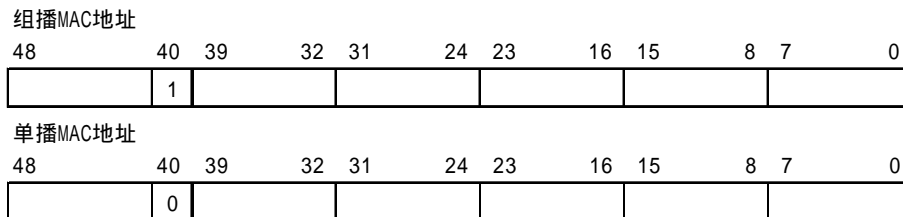
图 6-3 组播和单播 MAC 地址
