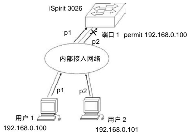
图 10-1 用户从绑定的端口接入网络
