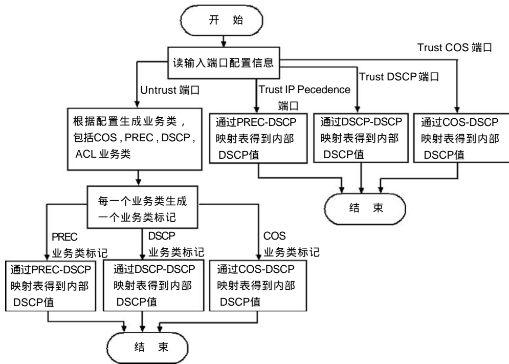
图 12-4 业务分类流程
