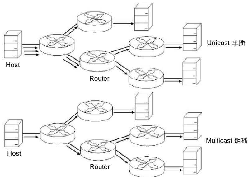
图 14-1 单播和组播方式传输信息比较
