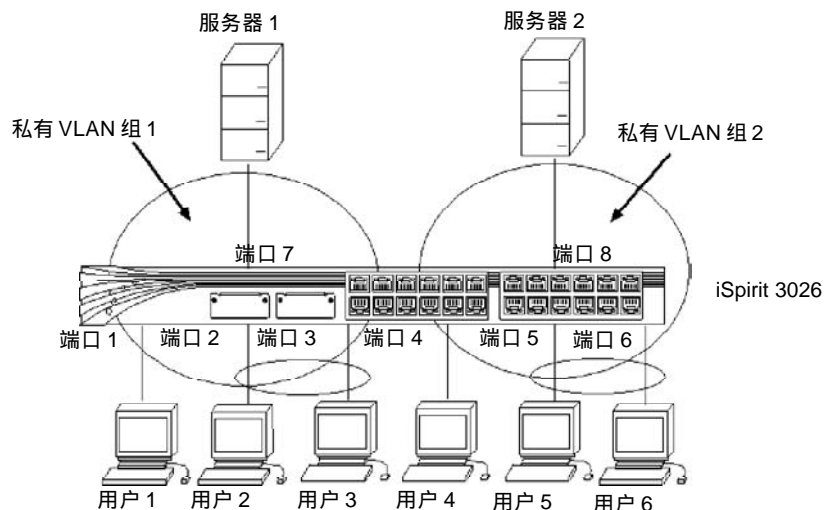
图 4-4 两个私有 VLAN 组
