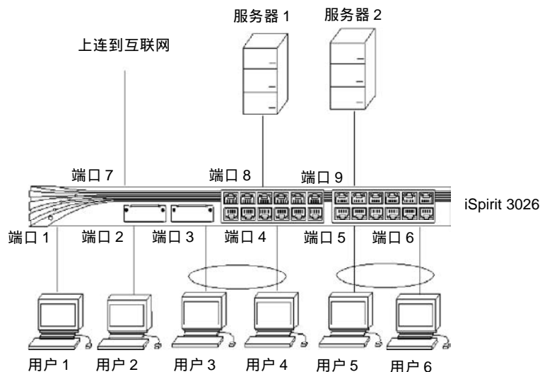
图 4-1 一个私有 VLAN 组
