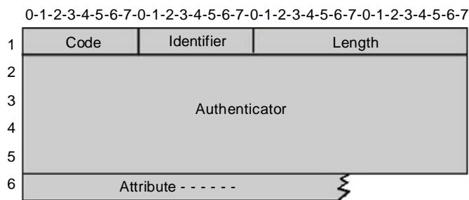
图 8-6 RADIUS 报文格式
