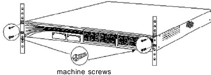
图 2-5 将交换机安装到机柜里
