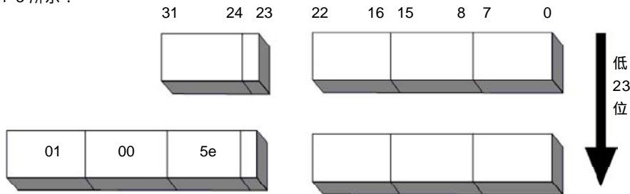
图 14-3 组播 IP 地址到组播 MAC 地址的转换
