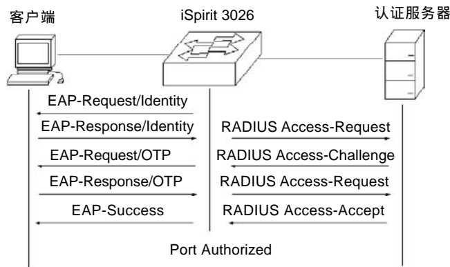
图 8-5 重新认证的协议交互
