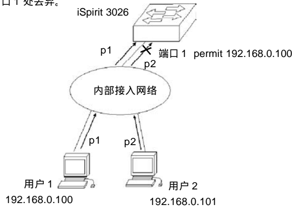
图 11-1 用户从 ACL 过滤的端口接入网络
