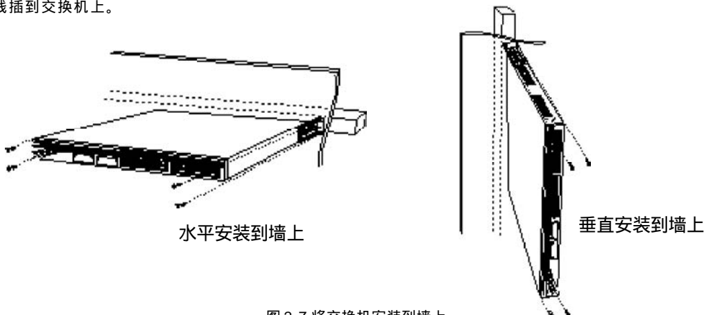
图 2-7 将交换机安装到墙上
