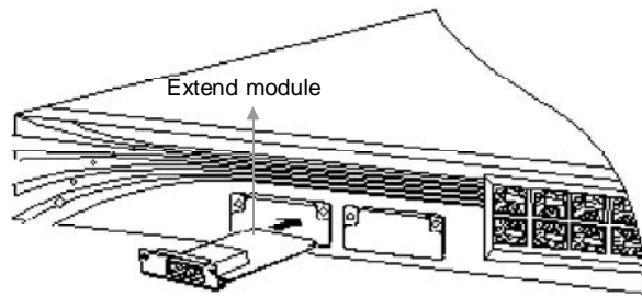
图 1-3 将模块插入交换机扩展模块插槽
