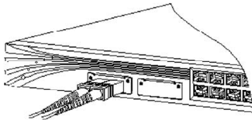
图 2-9 将 SC 接口插入光纤端口
