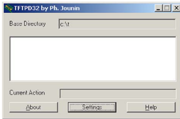
图 1-2 TFTPD32 界面图
