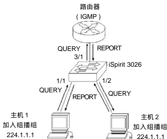
图 7-2 主机 1 和主机 2 加入组播组
