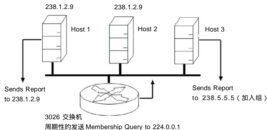
图 14-5 加入组的 IGMP 协议过程
