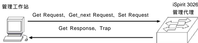
图 16-1 管理工作站和管理代理之间的 SNMP 协议交互
