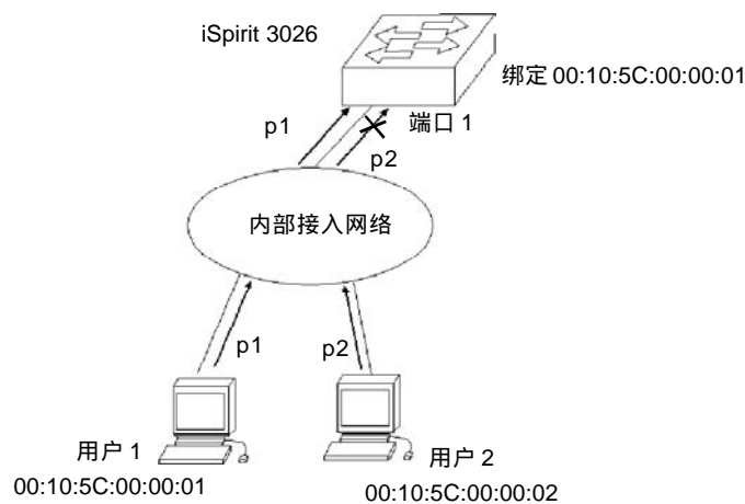
图 9-1 用户从绑定的端口接入网络
