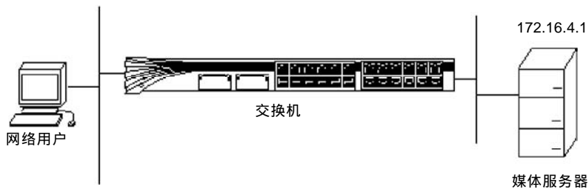
图 6-5 配置示例图
