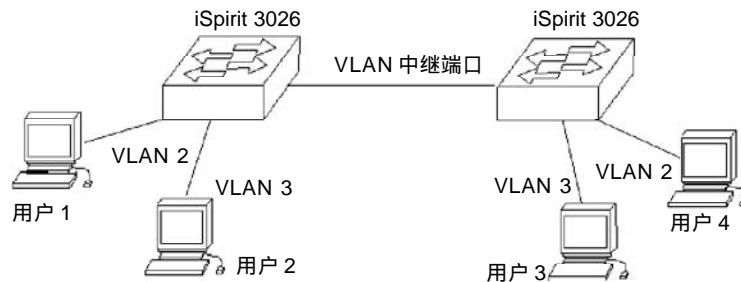
图 3-2 VLAN 中继端口
