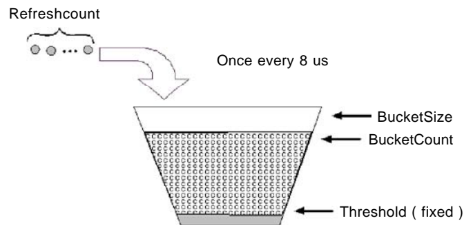
图 12-5 用于带宽限制的漏斗算法
