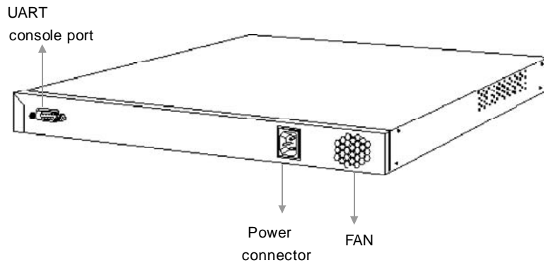
图 1-5 3026 交换机后面板
