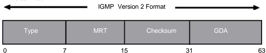
图 14-4 IGMPV2 的消息格式
