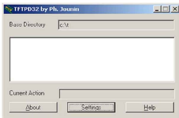
图 1-5 TFTPD32 界面图
