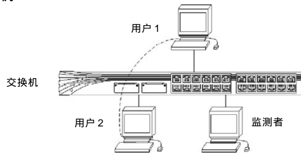
图 2-1 MIRROR 示例连接图
