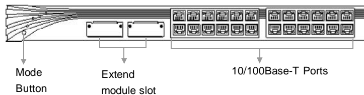
图 1-2 3026 交换机前面板
