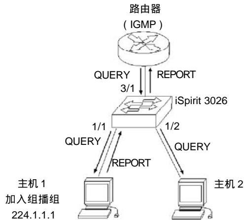
图 7-1 主机 1 加入组播组
