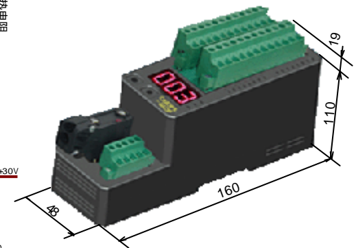
尺寸示意图
