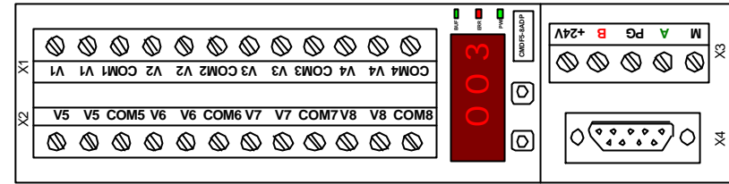
(图 1) CMD5-8ADP 端子示意图
