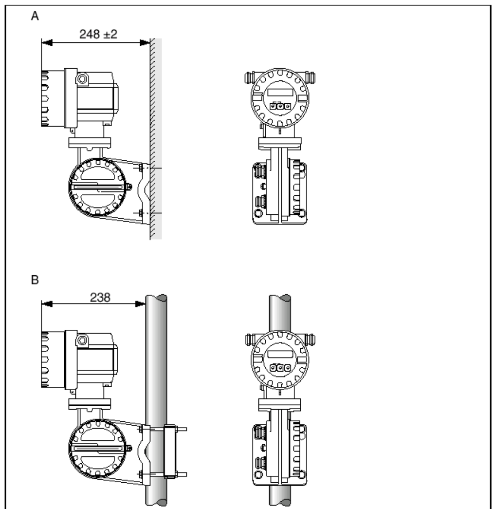
远方型变送器的安装
