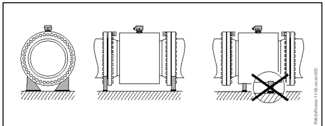
标称直径大 ( DN \geq 350 ) 的正确支撑
