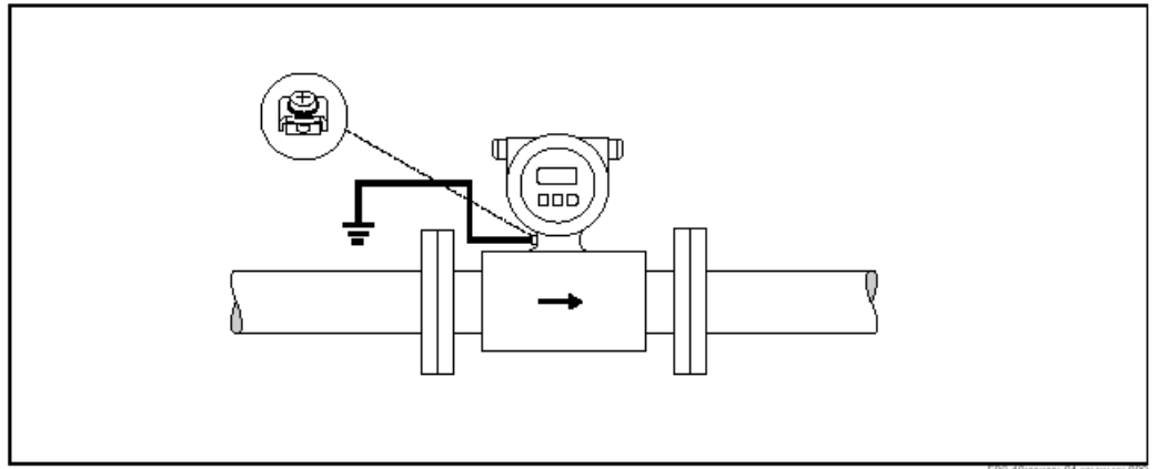
用变送器接地端子的等电位
