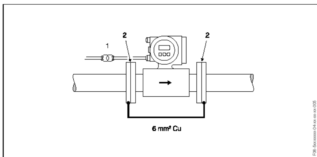
1 = 隔离变压器, 2 = 电气绝缘
