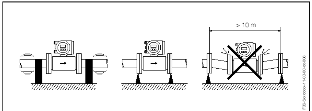
测量设备防止最大的方法
