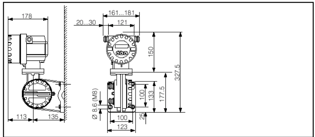
远方型 Promag 10 的尺寸
