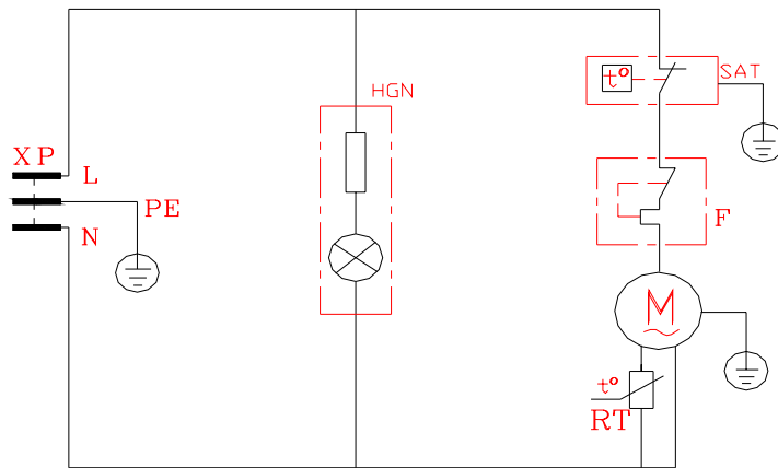
铭牌电路图
