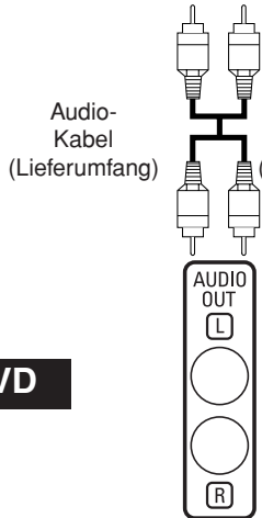
AUDIO OUT (Analog)
