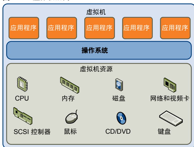
图 11-2 虚拟机隔离
