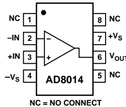
SOIC-8 (R)
