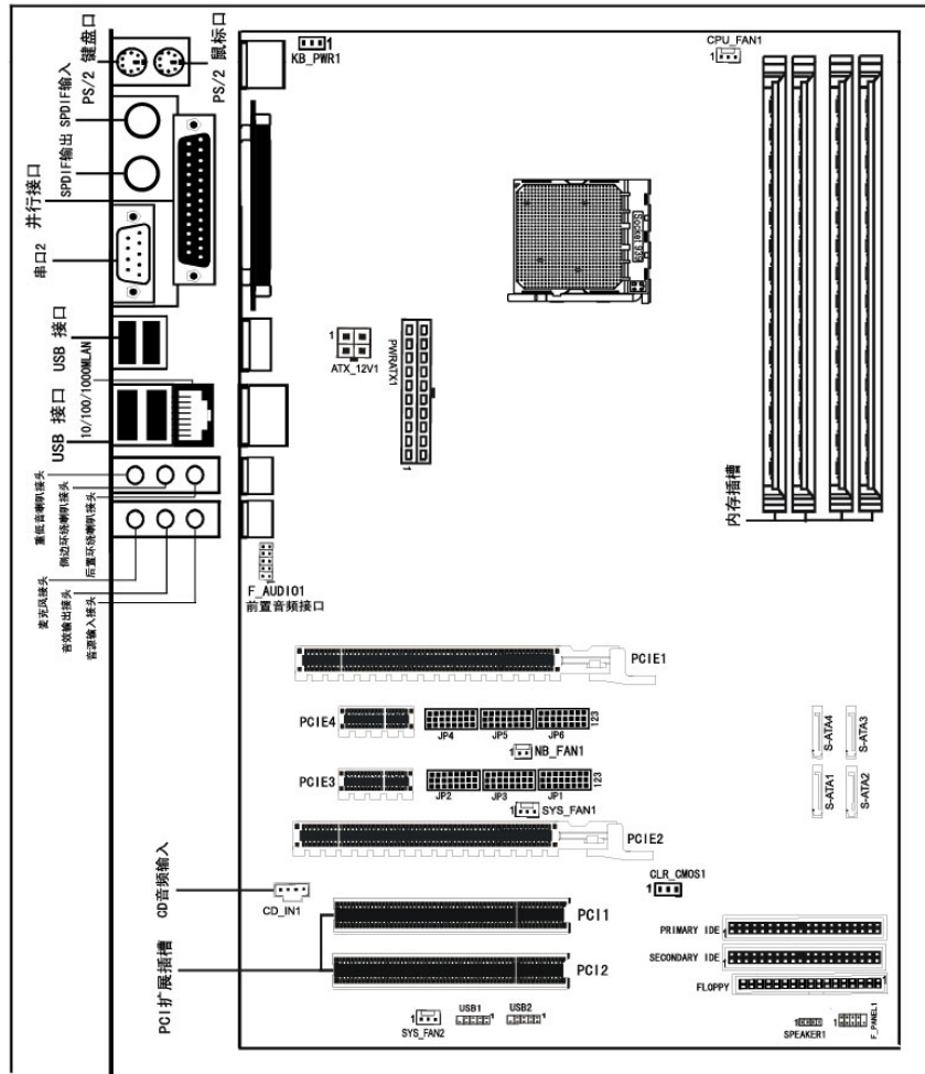
昂达 NF4SLI/NF4D 主板位图
