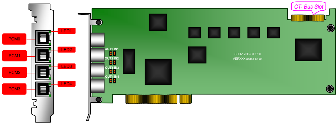
图 2-1 SHD-120D-CT/PCI 主板示意图 (左视图及正视图)
