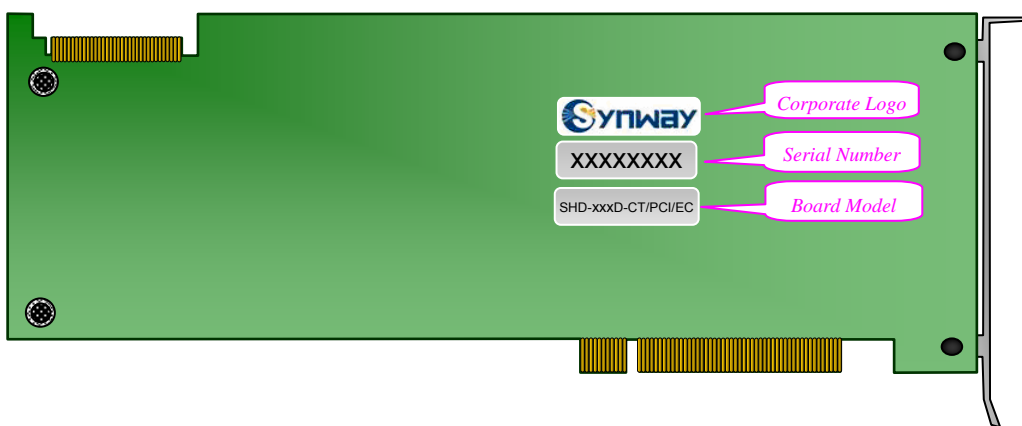
图 2-5 SHD-120/240D-CT/PCI 、 SHD-120/240D-CT/PCI/EC 主板后视图
