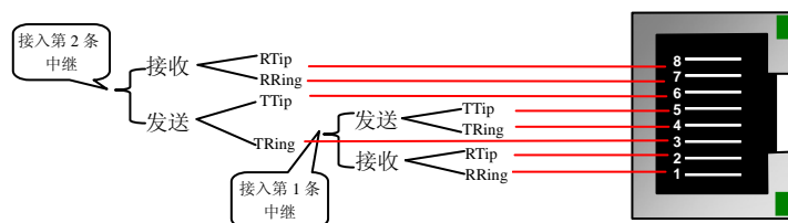
图 2-7 复用 RJ45 接口的引线图
