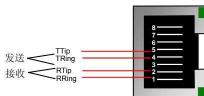
图 2-6 普通 RJ45 接口的引线图
