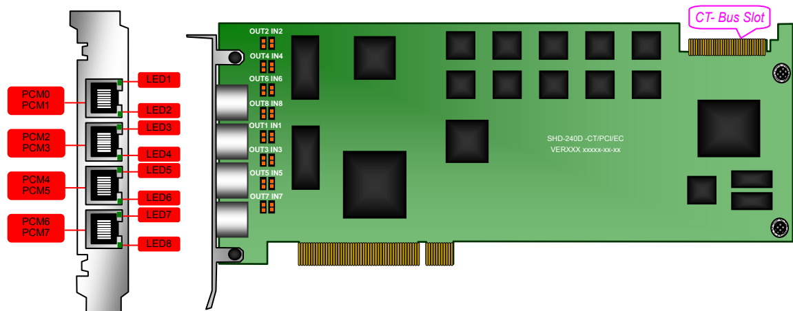
图 2-4 SHD-240D-CT/PCI/EC 主板示意图(左视图及正视图)
