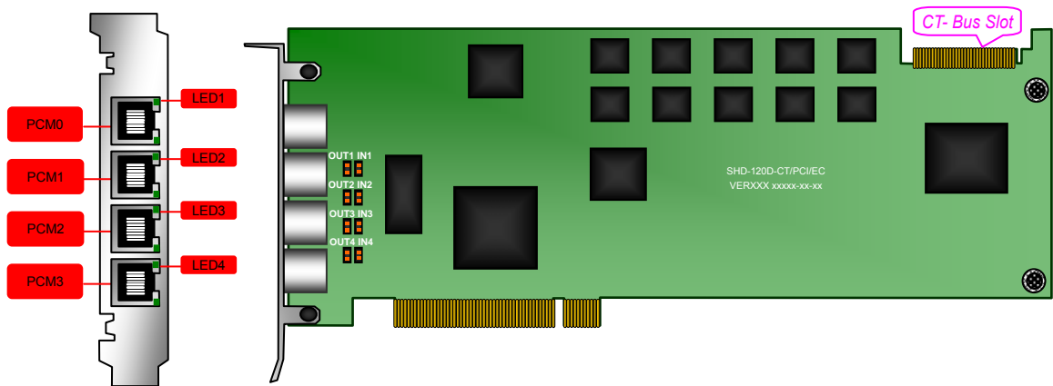
图 2-2 SHD-120D-CT/PCI/EC 主板示意图 (左视图及正视图)
