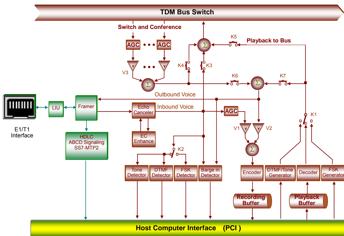
图 1-1 SHD-120/240D-CT/PCI/EC 型板卡工作原理图
