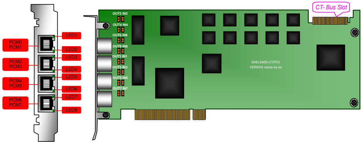
图 2-3 SHD-240D-CT/PCI 主板示意图（左视图及正视图）
