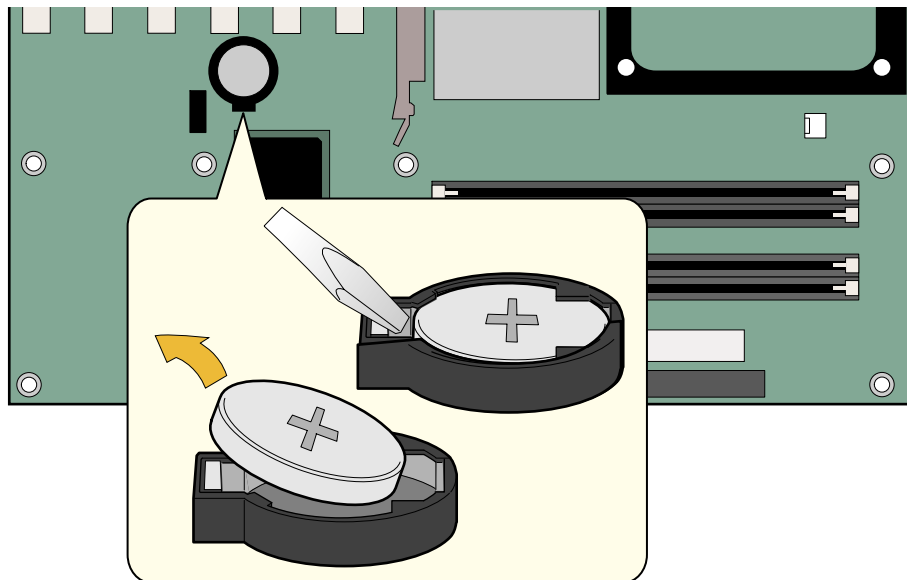
图 17. 拆卸电池
