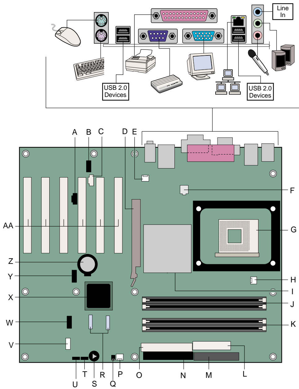
图 1. 桌面主板 D865GBF 组件
