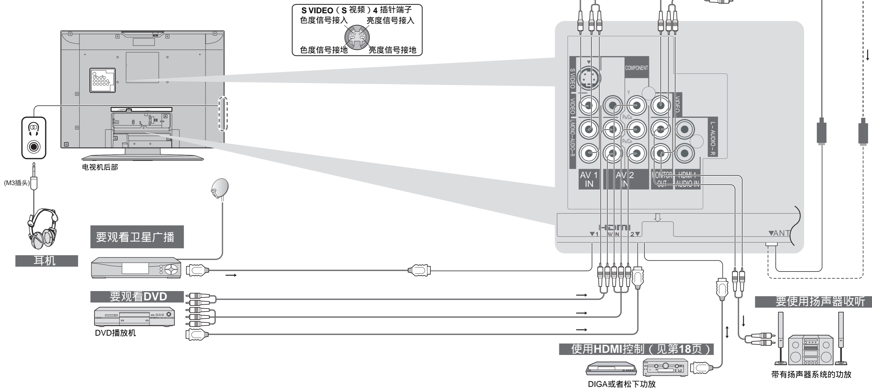
连接至每一端子的可连接设备类型
