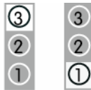
2-3闭合清除CMOS 1-2闭合正常 跳线丝印处有白色标记的地方为第一针脚
