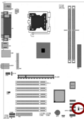
2-3闭合清除CMOS 1-2闭合正常 跳线丝印处有白色标记的地方为第一针脚
