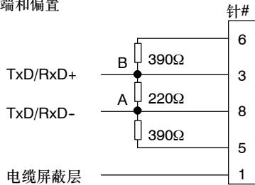
图7-22 网络电缆的偏置和终端
