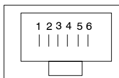
图A-30 RJ11插座的视图
