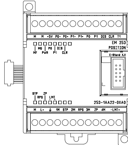
图9-9 EM253位控模块
