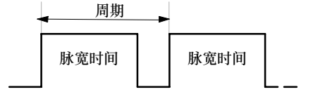
图9-1 脉宽调制（PWM）
