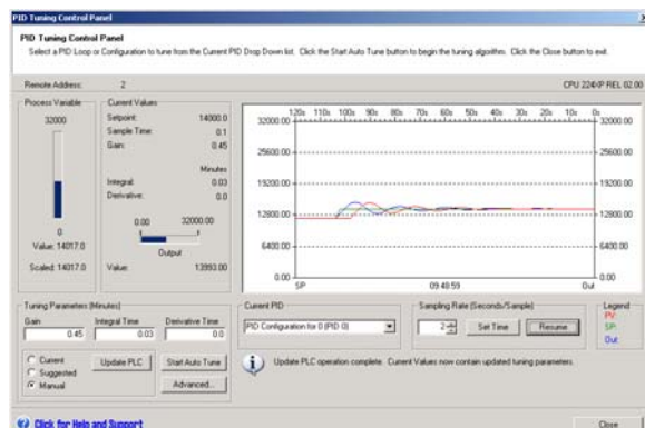
图15-4 对设定值变化的响应
