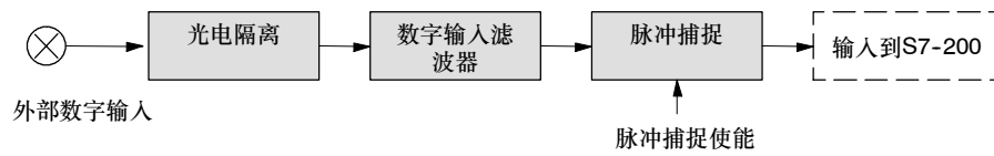
图4-26 数字量输入电路
