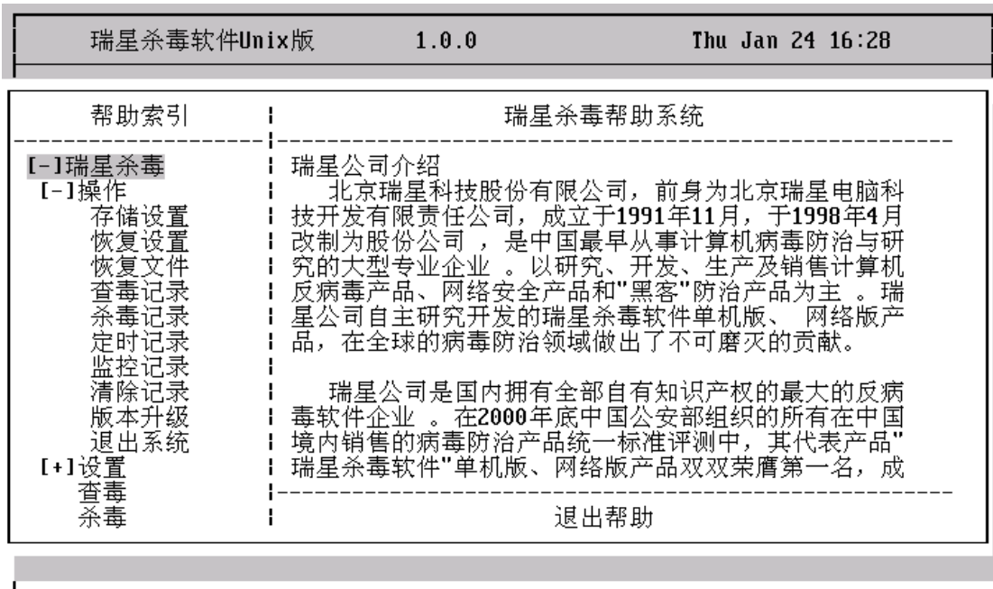
图 12 帮助菜单
