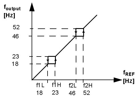
图 7 危险频率设定示例。在 18 - 23Hz, 46 - 52Hz 之间，风机摇摆不定
