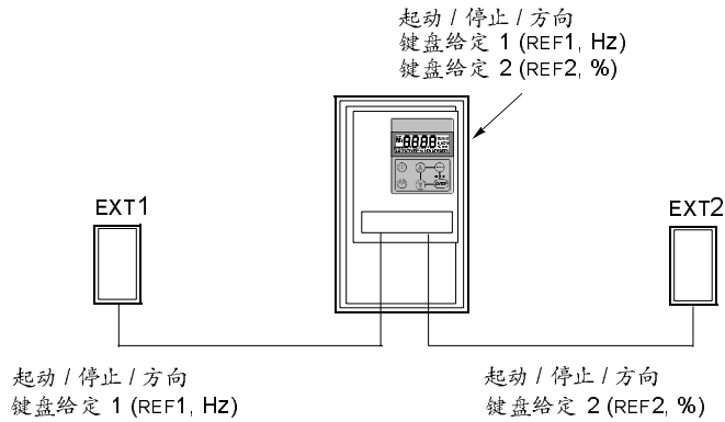
图 23 控制方式
