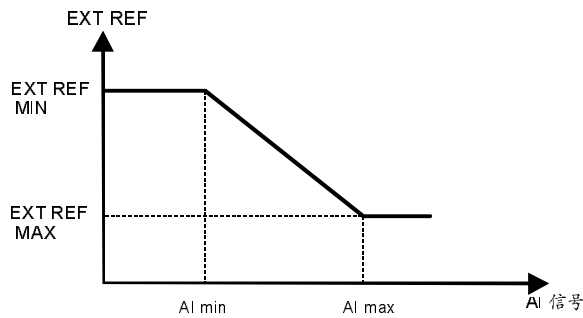
图 3 设定外部给定的低限和高限。依选择的 AI 通道而有所不同, AI 信号的范围由参数 1301 和 1302 或 1304 和 1305 确定。
