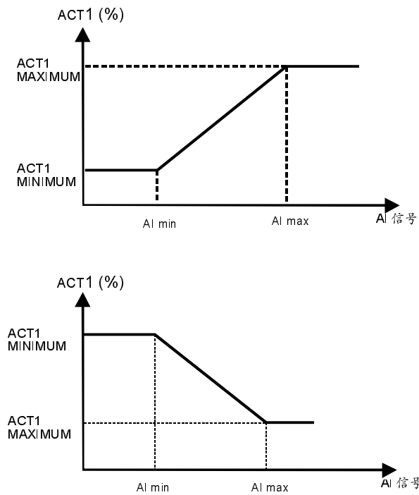
图 16 实际值换算。AI 信号变换范围，由参数 1301，1302 或 1304，1305 决定。
