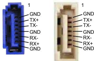
SATA_1/2/3/4/5
