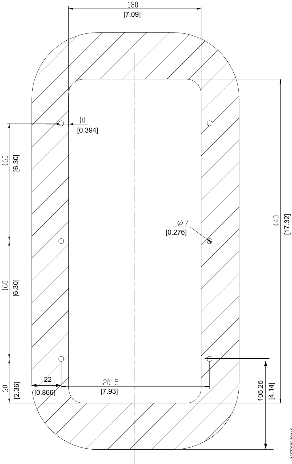
外形尺寸图
