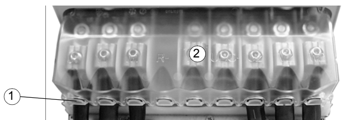
电缆接线端子安装示意图
