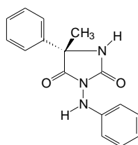
RPA 410193
