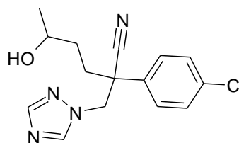
RH-9090
