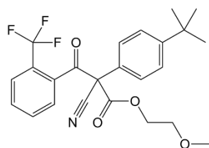
Cyflumetofen
