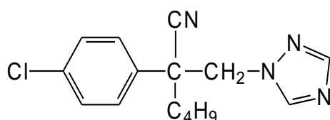
Myclobutanil
