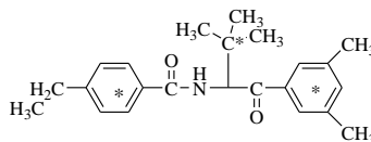
Tebufenozide
