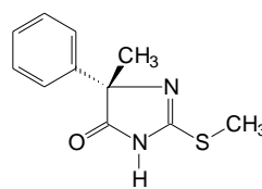
RPA412708
